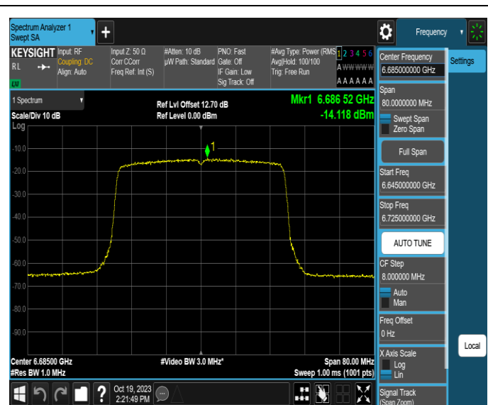
11AX40MIMO-Ant4-6685-PASS
