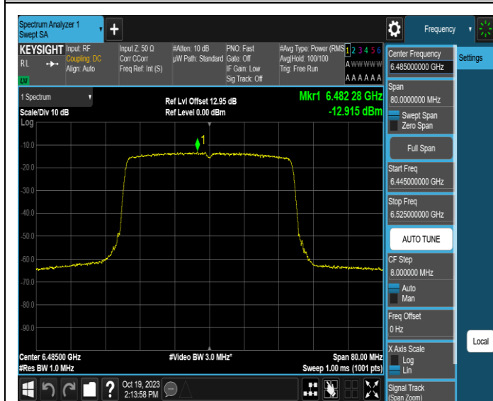
11AX40MIMO-Ant1-6485-PASS
