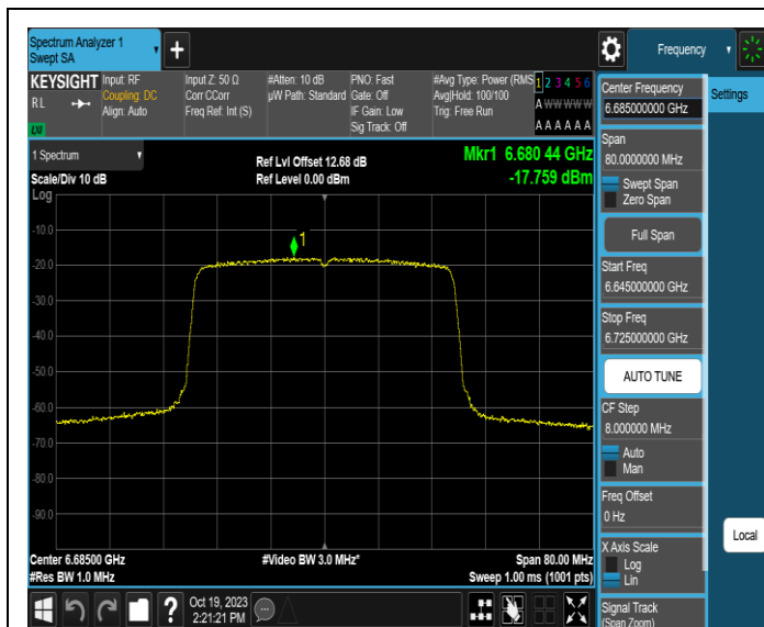
11AX40MIMO-Ant3-6685-PASS
