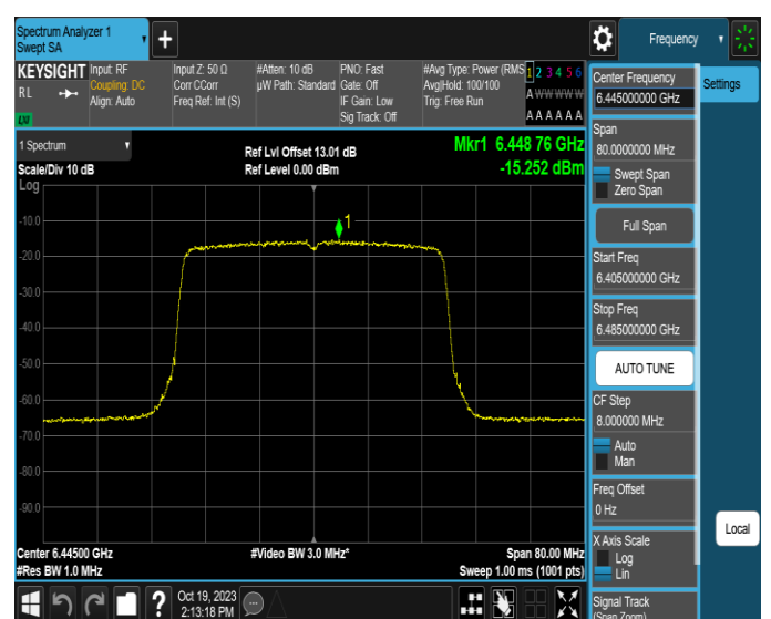
11AX40MIMO-Ant4-6445-PASS
