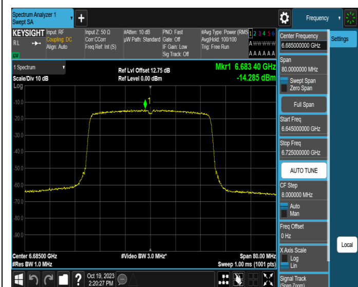
11AX40MIMO-Ant1-6685-PASS
