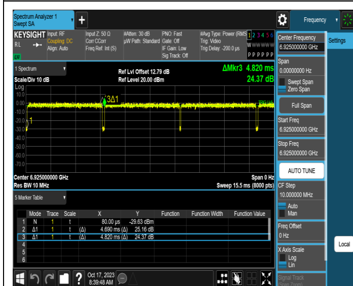
NTNV-11AX40MIMO-Ant1-6925
