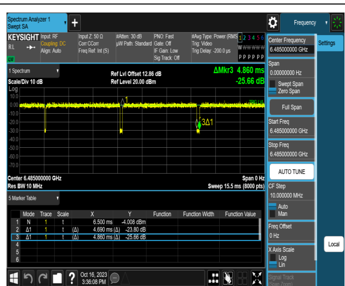
NTNV-11AX40MIMO-Ant4-6485
