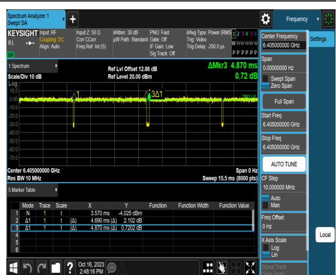
NTNV-11AX40MIMO-Ant4-6405
