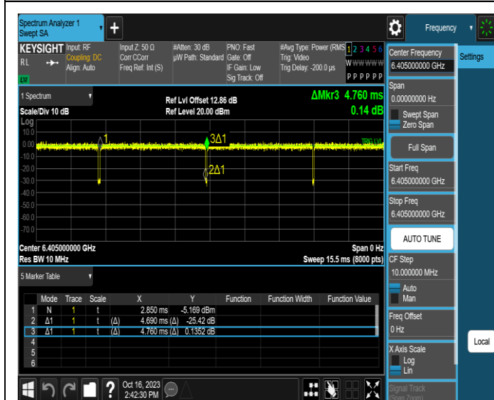
NTNV-11AX40MIMO-Ant3-6405
