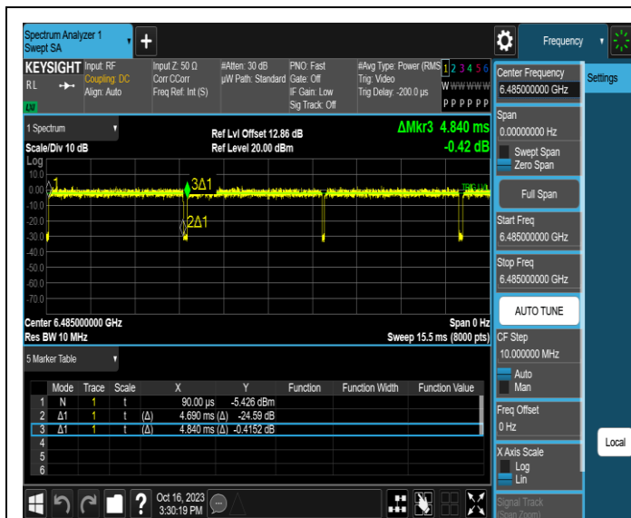
NTNV-11AX40MIMO-Ant3-6485
