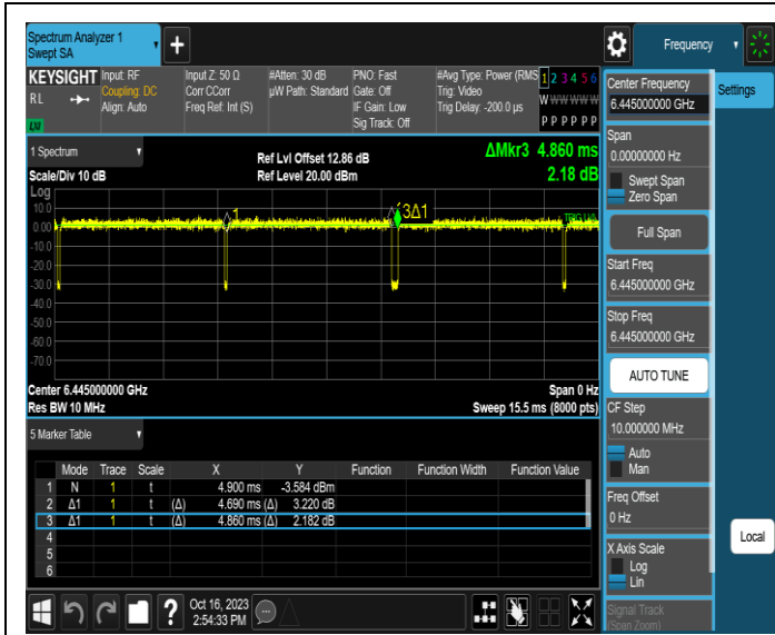
NTNV-11AX40MIMO-Ant1-6445
