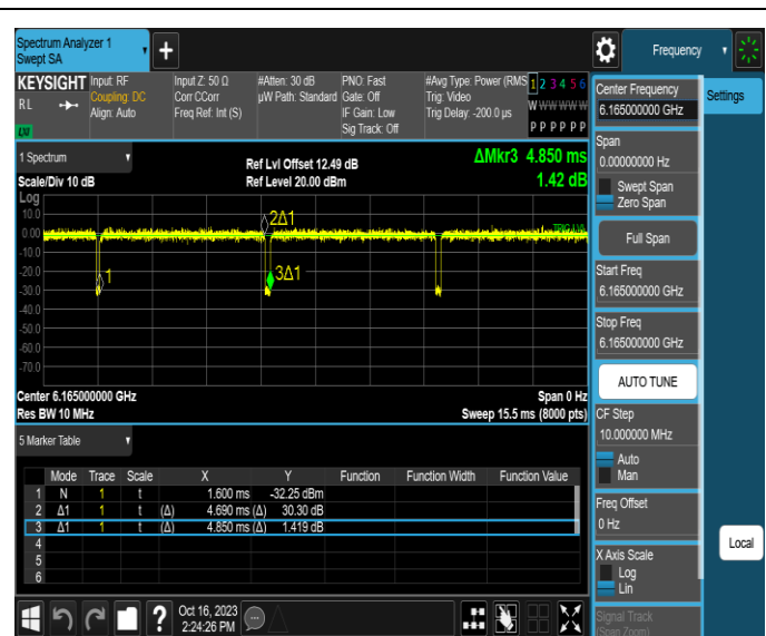
NTNV-11AX40MIMO-Ant4-6165
