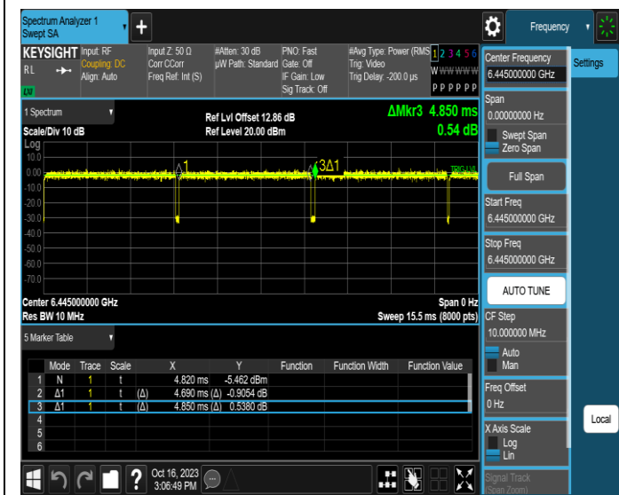
NTNV-11AX40MIMO-Ant3-6445
