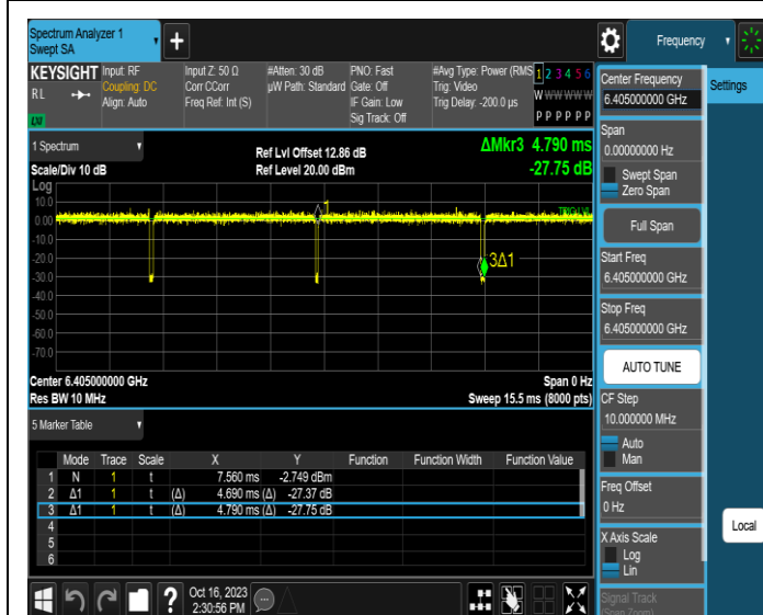
NTNV-11AX40MIMO-Ant1-6405
