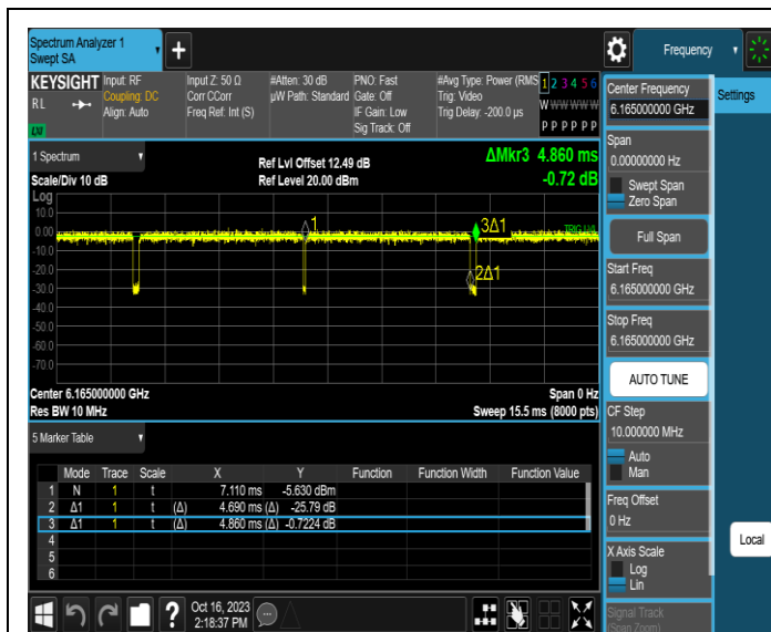
NTNV-11AX40MIMO-Ant3-6165
