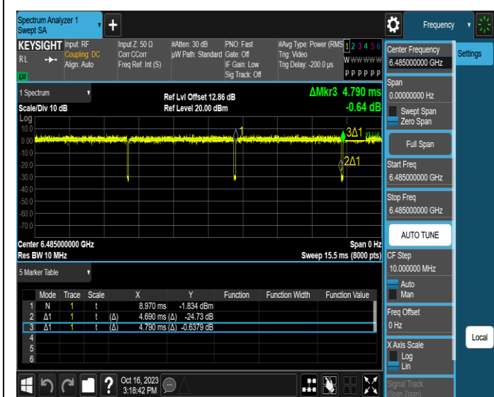
NTNV-11AX40MIMO-Ant1-6485
