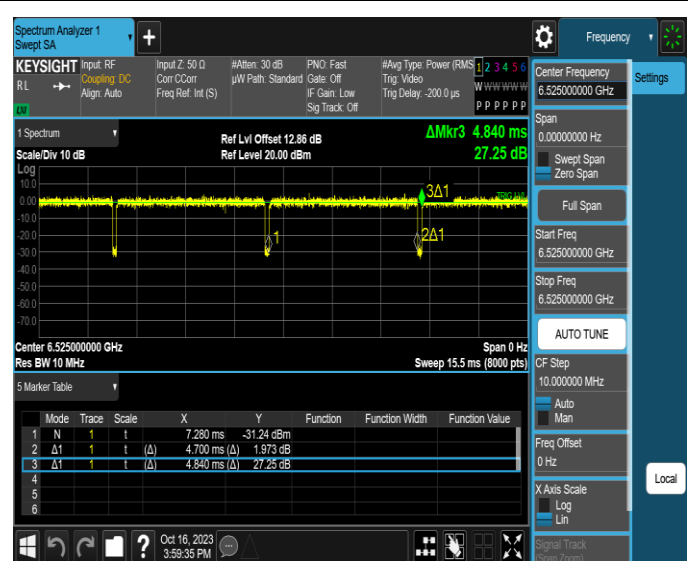
NTNV-11AX40MIMO-Ant4-6525
