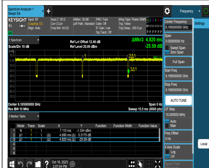
NTNV-11AX40MIMO-Ant1-6165
