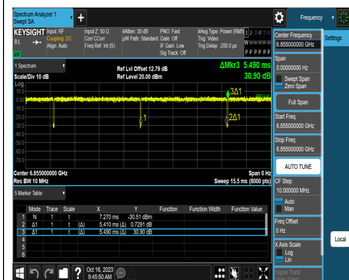
NTNV-11AX20MIMO-Ant3-6855
