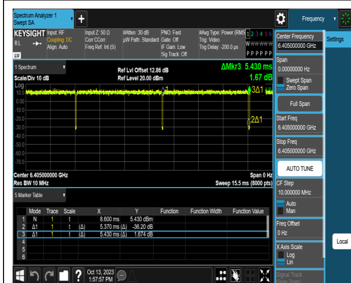
NTNV-11AX40SISO-Ant1-6405
