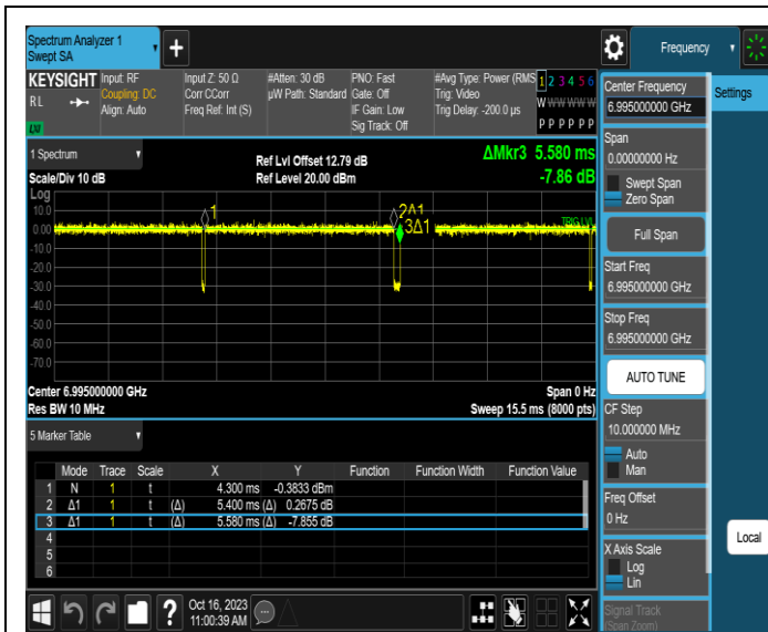
NTNV-11AX20MIMO-Ant1-6995
