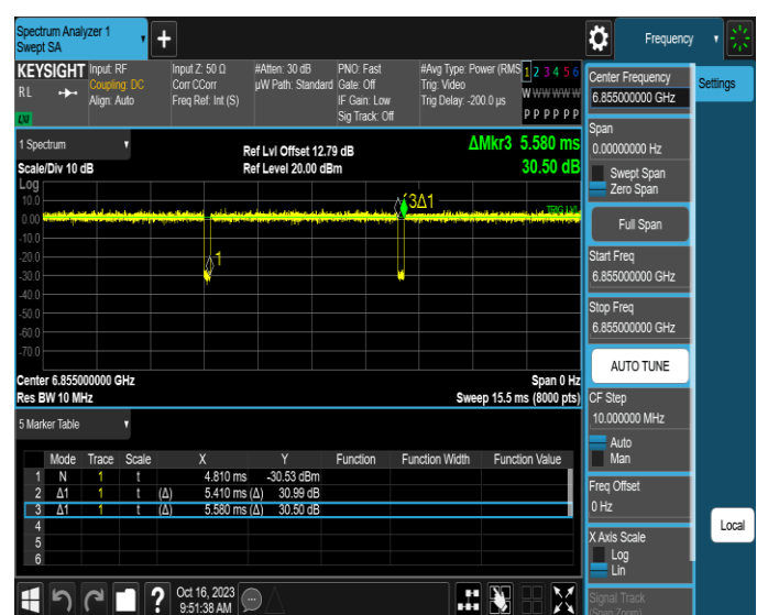
NTNV-11AX20MIMO-Ant4-6855
