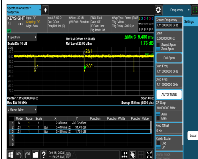
NTNV-11AX20MIMO-Ant1-7115
