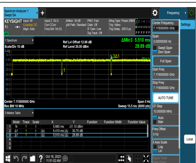
NTNV-11AX20MIMO-Ant4-7115
