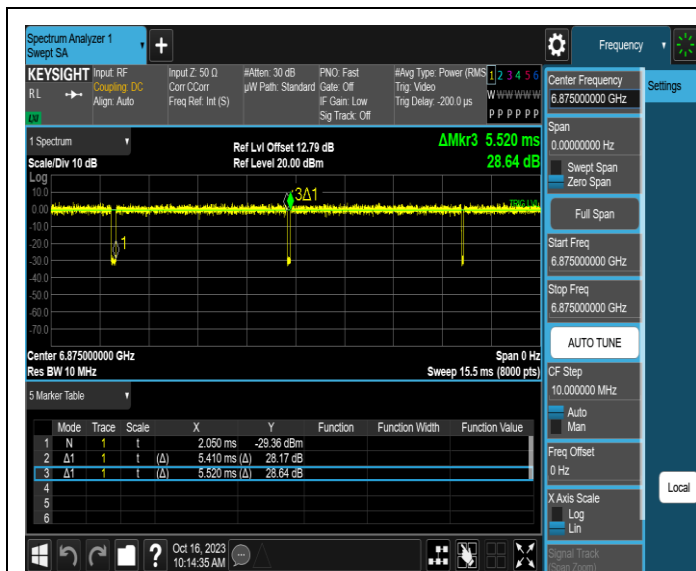
NTNV-11AX20MIMO-Ant3-6875
