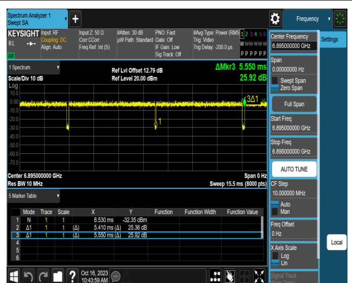
NTNV-11AX20MIMO-Ant4-6895
