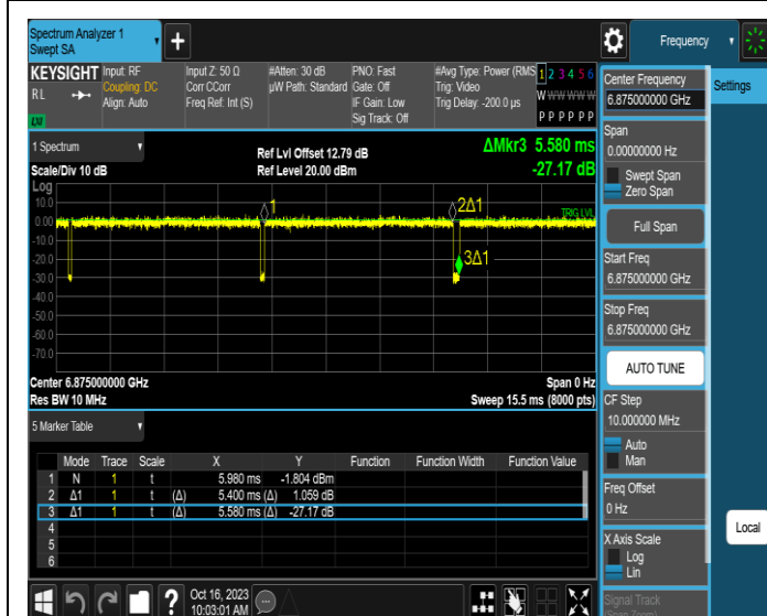
NTNV-11AX20MIMO-Ant1-6875
