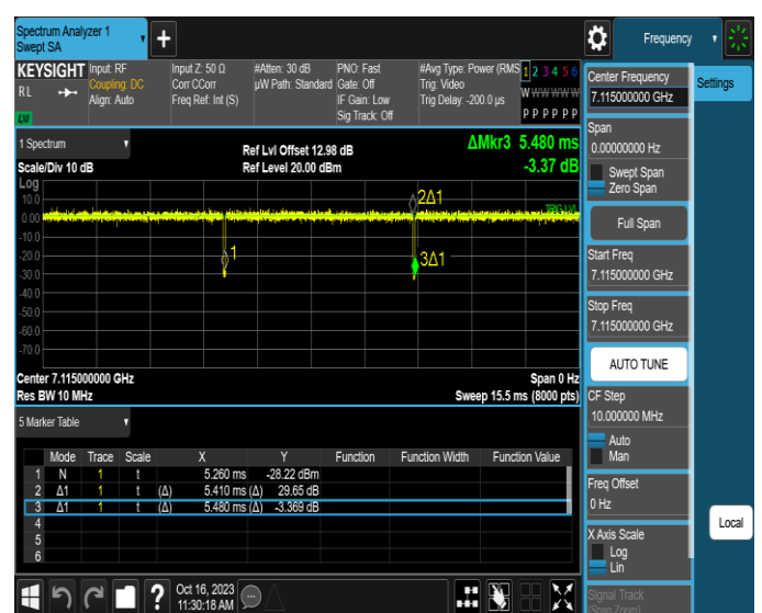
NTNV-11AX20MIMO-Ant2-7115
