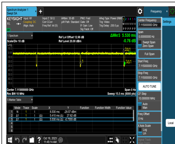
NTNV-11AX20MIMO-Ant3-7115
