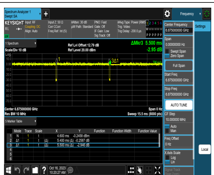
NTNV-11AX20MIMO-Ant4-6875
