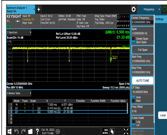
NTNV-11AX20MIMO-Ant1-6535
