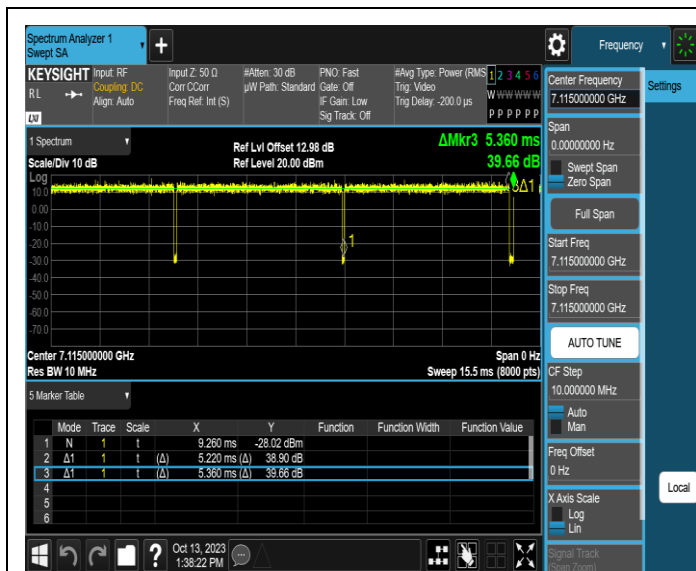
NTNV-11AX20SISO-Ant1-7115
