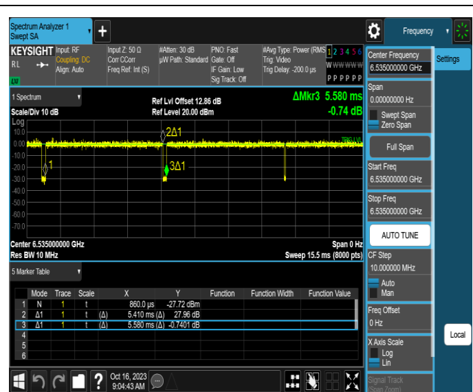
NTNV-11AX20MIMO-Ant4-6535
