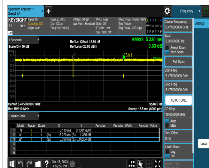
NTNV-11AX20MIMO-Ant3-6475
