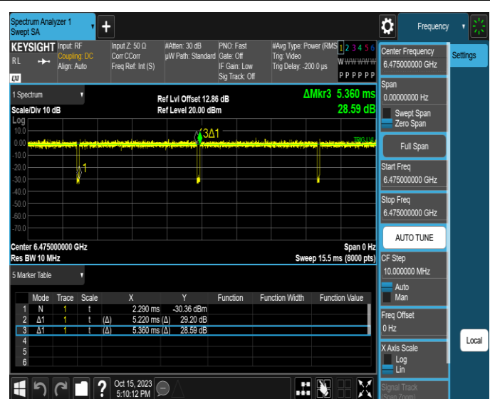
NTNV-11AX20MIMO-Ant4-6475
