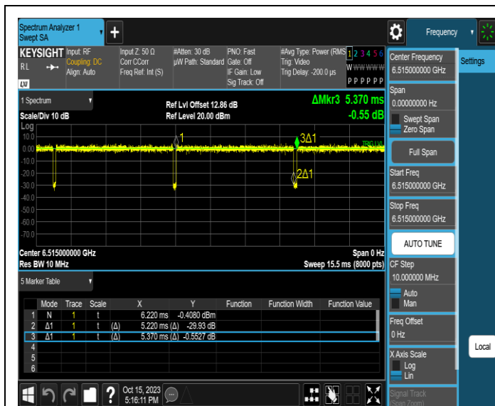
NTNV-11AX20MIMO-Ant1-6515
