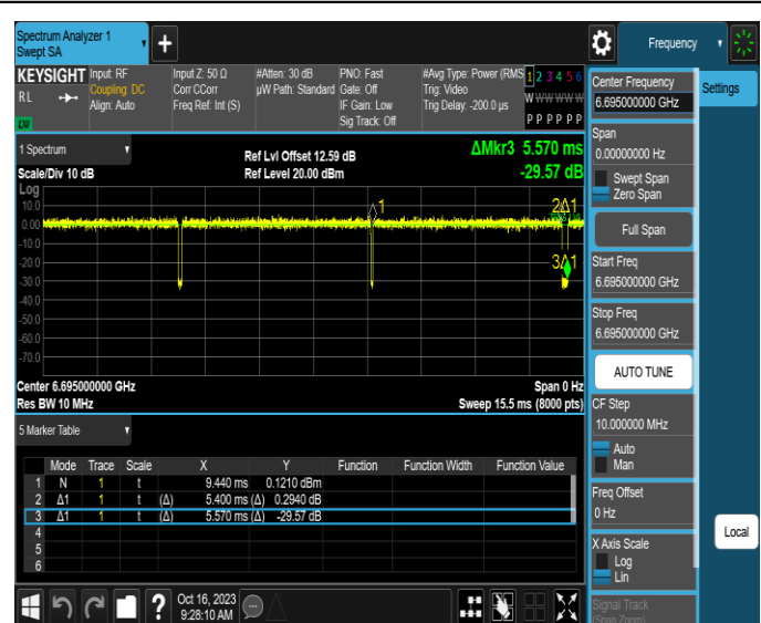
NTNV-11AX20MIMO-Ant4-6695
