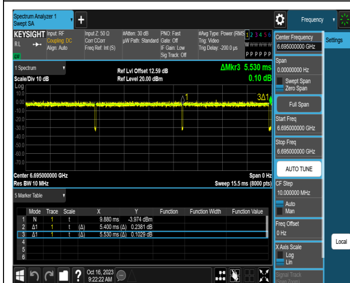
NTNV-11AX20MIMO-Ant3-6695
