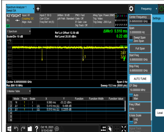
NTNV-11AX20MIMO-Ant1-6695
