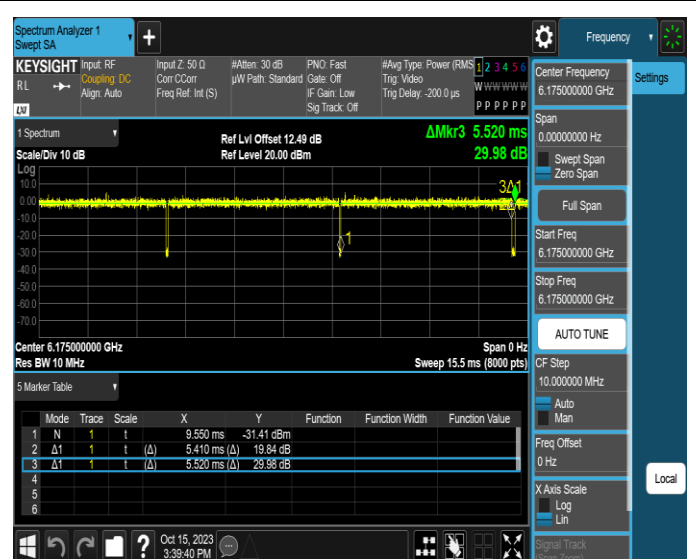
NTNV-11AX20MIMO-Ant4-6175
