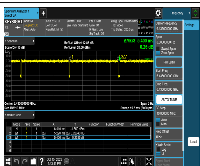
NTNV-11AX20MIMO-Ant4-6435
