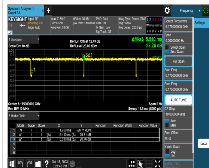
NTNV-11AX20MIMO-Ant3-6175
