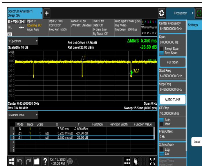
NTNV-11AX20MIMO-Ant3-6435
