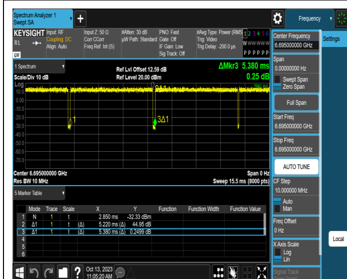
NTNV-11AX20SISO-Ant1-6695
