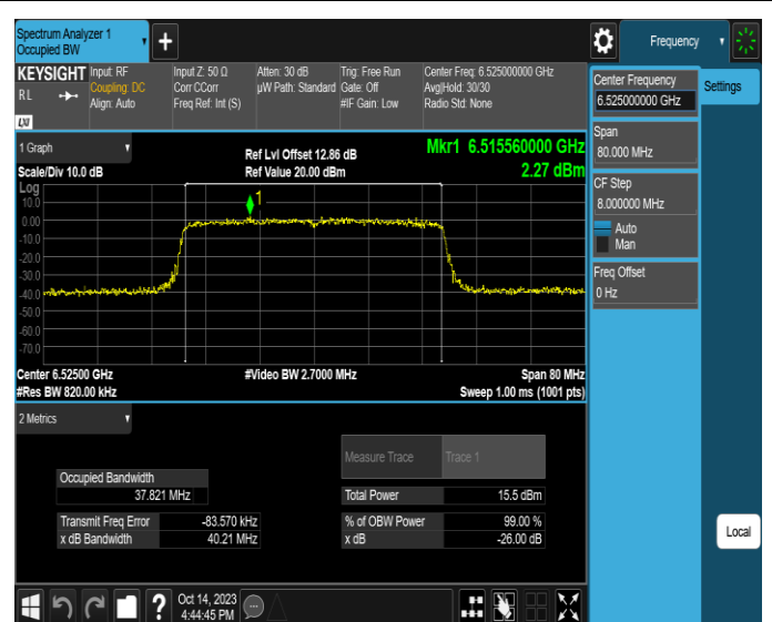
11AX40ISO-Ant4-6525
