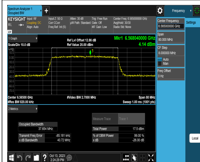
11AX40ISO-Ant1-6565
