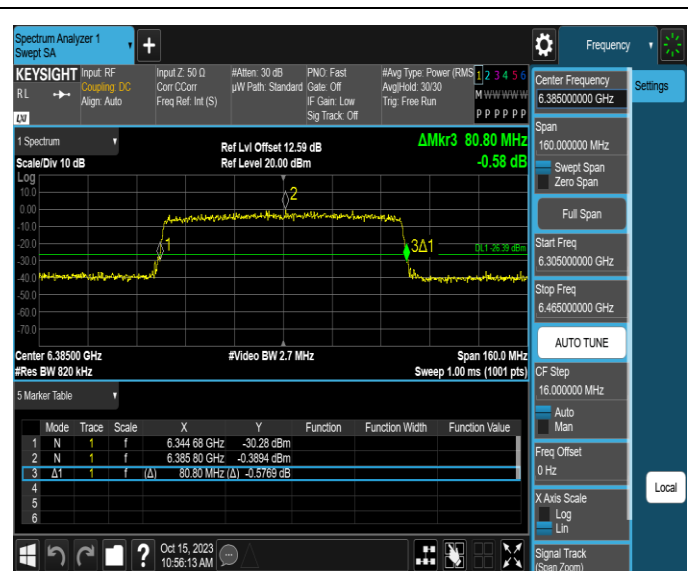
11AX80SISO-Ant4-6385
