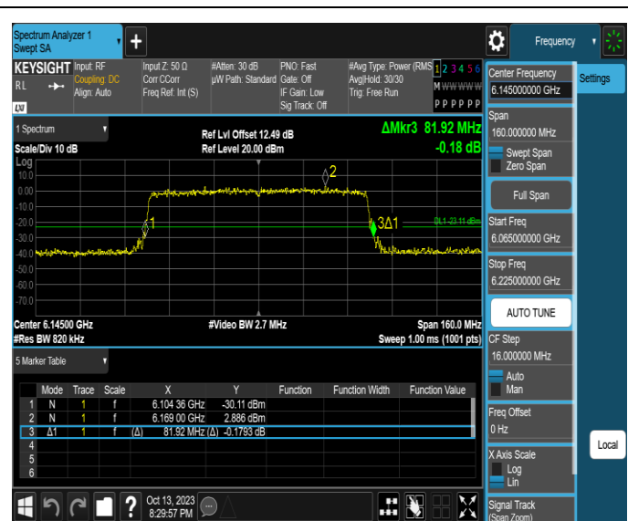
11AX80SISO-Ant2-6145
