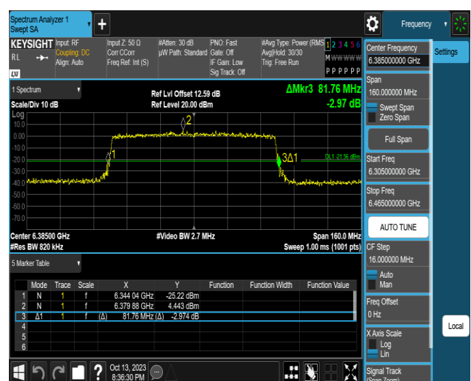
11AX80SISO-Ant2-6385
