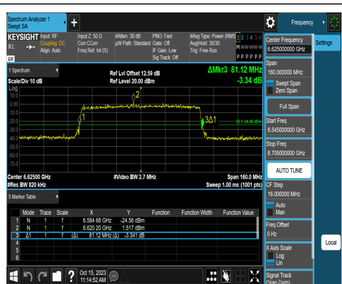
11AX80SISO-Ant4-6625
