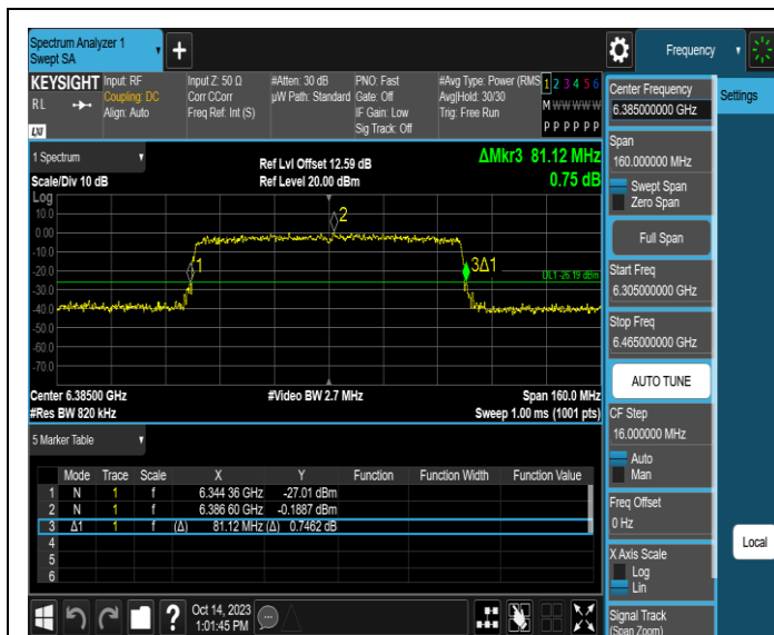
11AX80SISO-Ant3-6385
