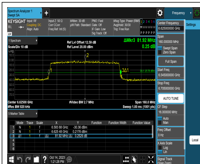
11AX80SISO-Ant3-6625
