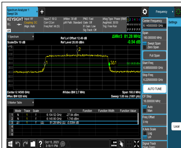
11AX80SISO-Ant1-6145
