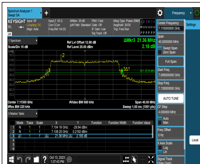
11AX20SISO-Ant1-7115
