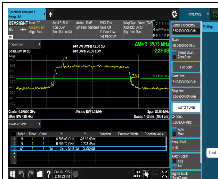
11AX40ISO-Ant1-6525
