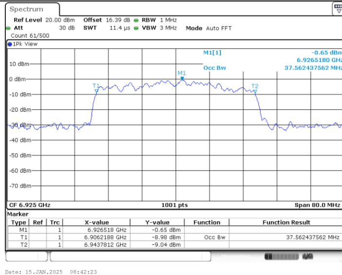
11AX40MIMO_Ant2_6925
