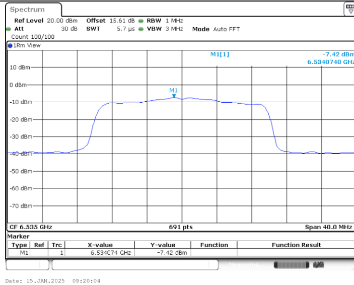
11AX20MIMO_Ant2_6535
