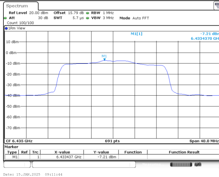
11AX20MIMO_Ant2_6435
