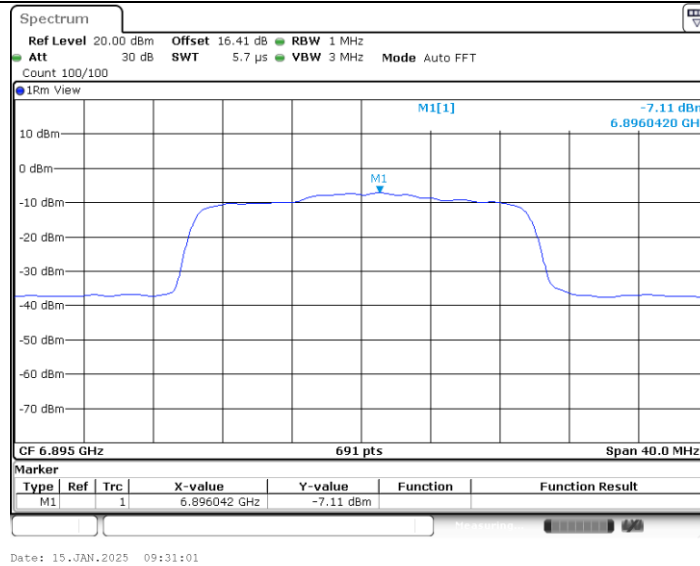
11AX20MIMO_Ant2_6895
