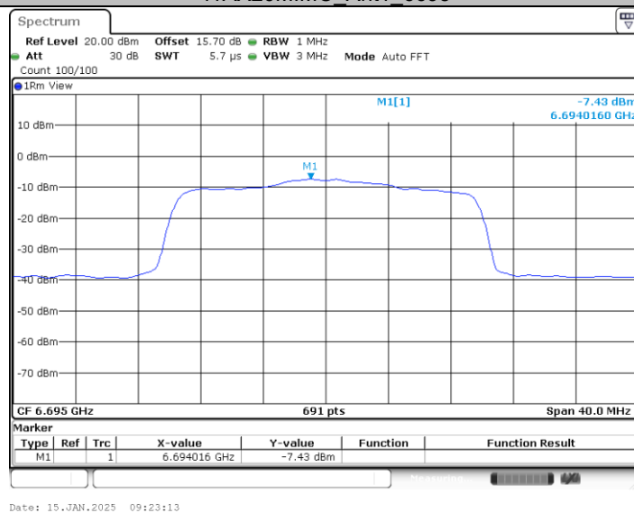
11AX20MIMO_Ant2_6695
