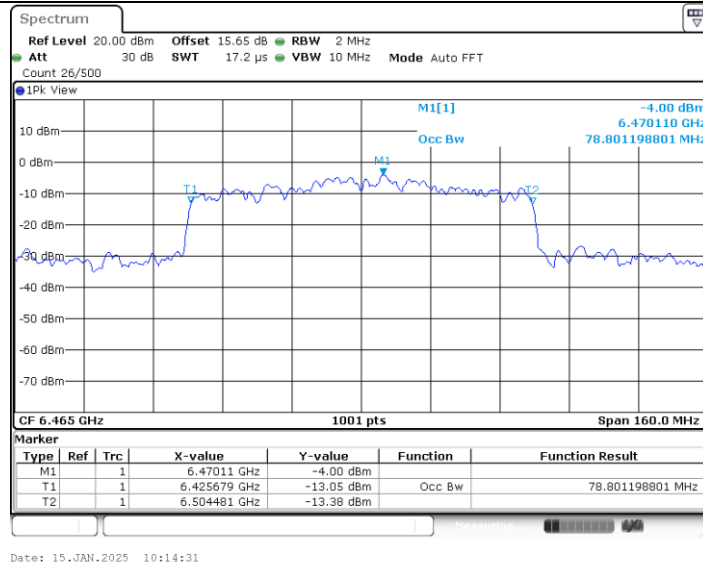
11AX80MIMO_Ant2_6465
