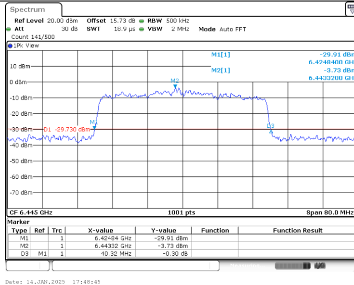
11AX40MIMO_Ant2_6445
