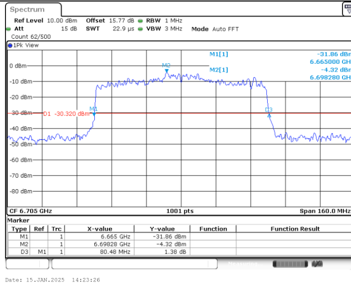
11AX80MIMO_Ant2_6705
