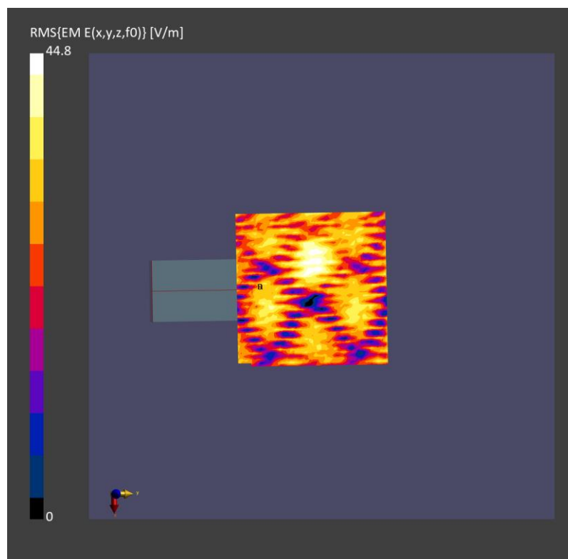
Fig. 2 WLAN 6GHz PD
