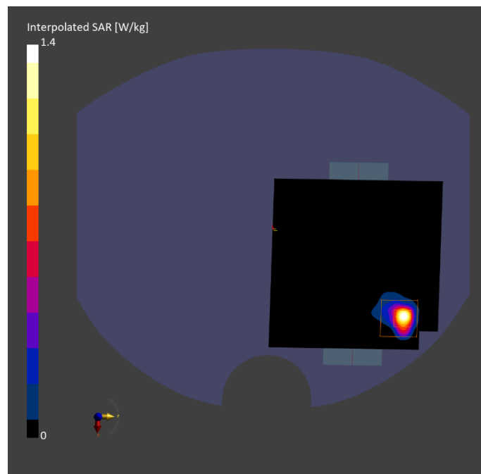
Fig. 1 WLAN 6GHz Body
