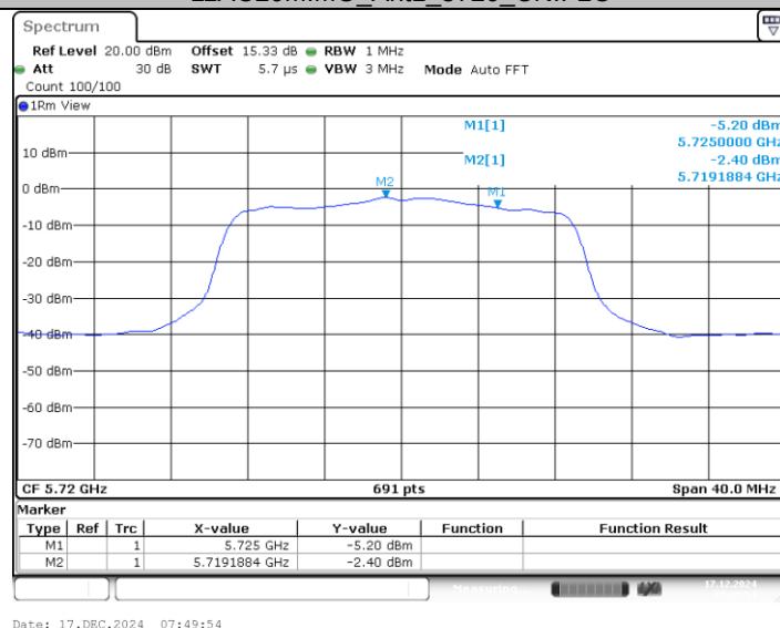
11AC20MIMO_Ant2_5720_UNII-2C
