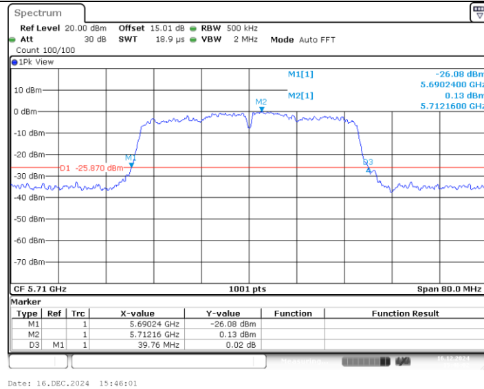
11N40MIMO_Ant2_5710
