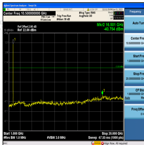
Band4-20MHz-QPSK-20050-100RB#0-Range2:1000~20000MHz
