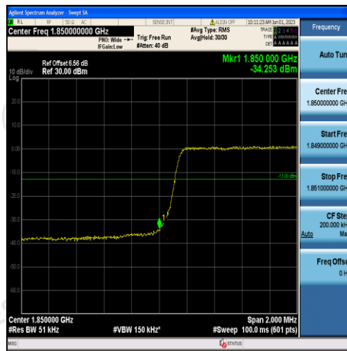
Band2-3MHz-16QAM-18615-15RB#0
