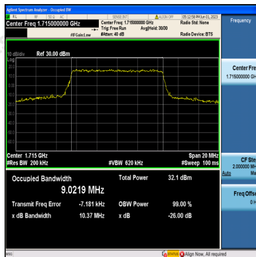
Band66-10MHz-QPSK-132022-50RB#0-9.0219
