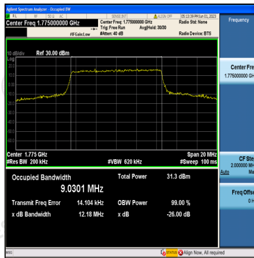
Band66-10MHz-QPSK-132622-50RB#0-9.0301
