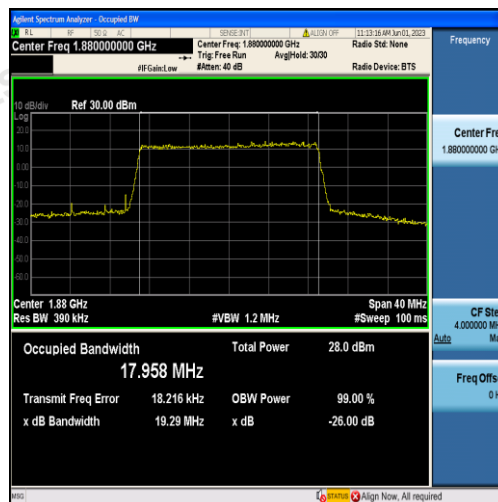
Band2-20MHz-QPSK-18900-100RB#0-17.958
