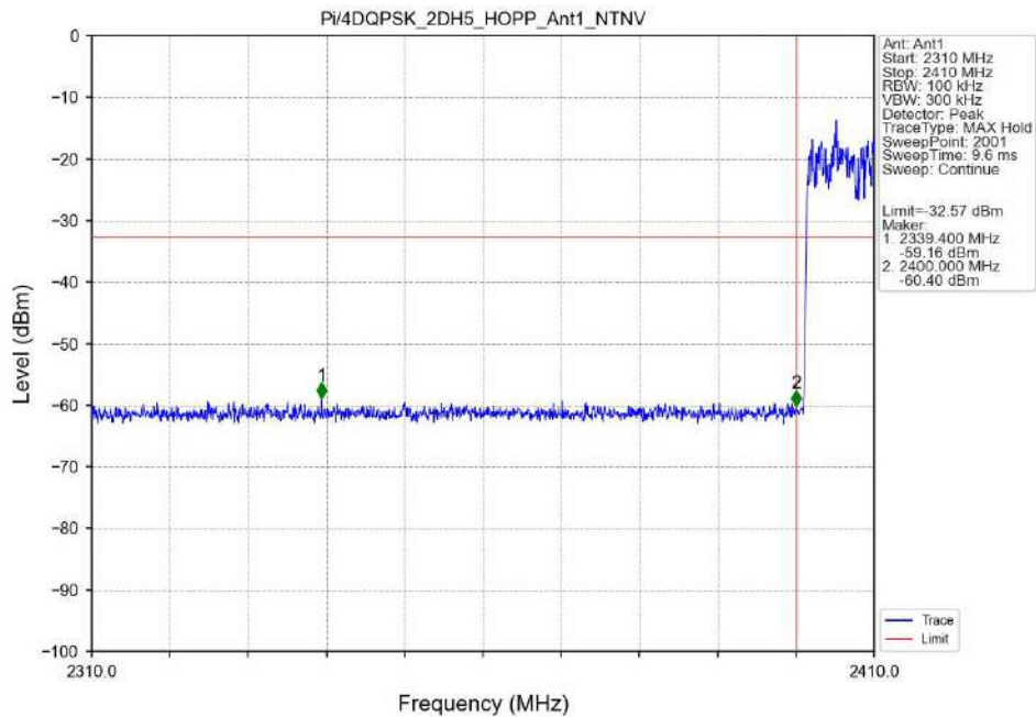
Pi/4DQPSK_2DH5_HOPP_Ant1_NTNV
