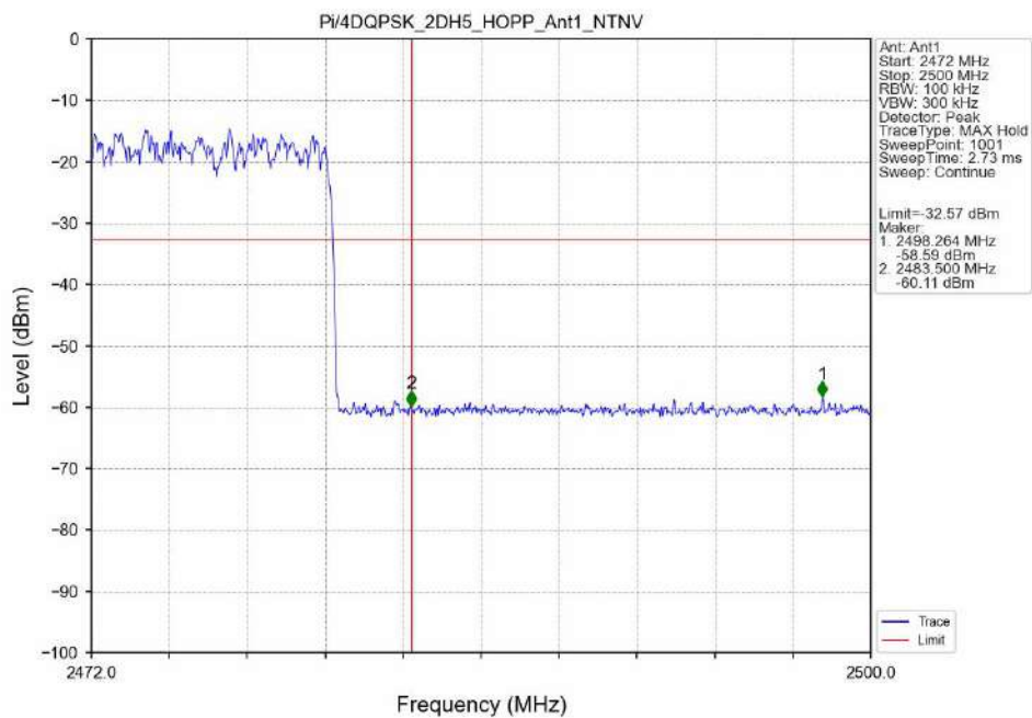
Pi/4DQPSK_2DH5_HOPP_Ant1_NTNV
