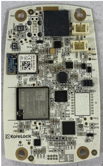
PCBA Top side
