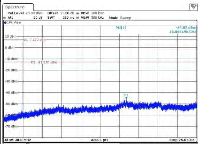
Tx 2402MHz / 30MHz~25GHz (down 20dBc)
