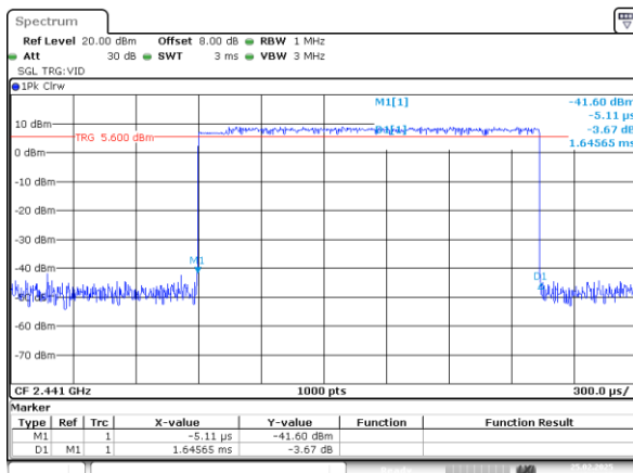
2DH3_Hopping 1.646ms
