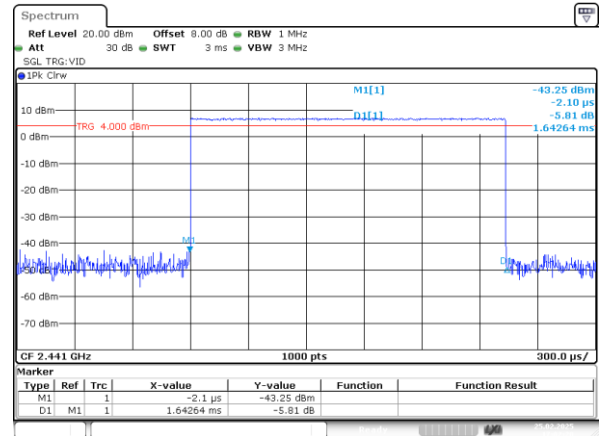
DH3_Hopping 1.643ms
