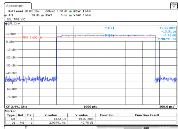
2DH5_Hopping 2.908ms
