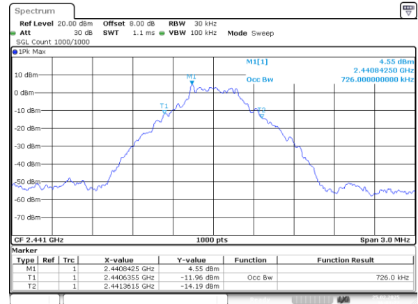
DH1_Middle 0.726MHz
