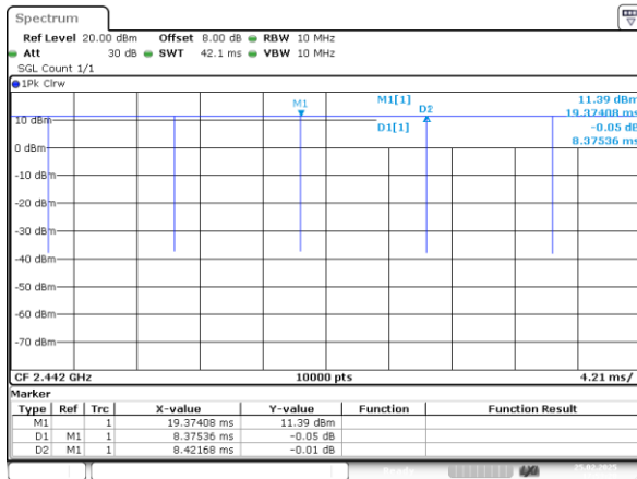
802.11b_2442MHz_Chain 0
