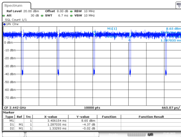
802.11n20_2442MHz_Chain 0
