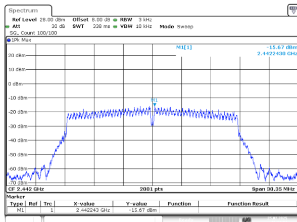
802.11n20_2442MHz_Chain 1
