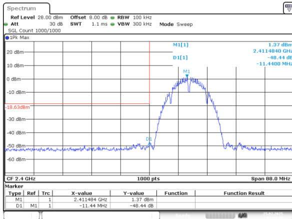
802.11b_2412MHz_Chain 1
