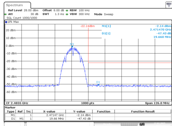
802.11b_2472MHz_Chain 0
