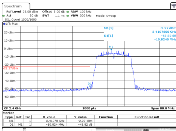
802.11n20_2412MHz_Chain 1
