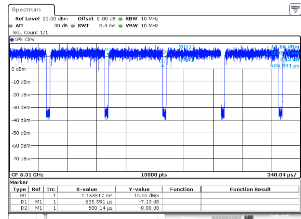
802.11n40_5310MHz_Chain 1
