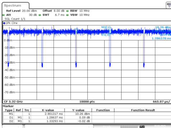
802.11n20_5320MHz_Chain 0
