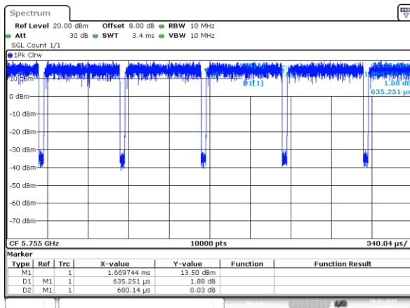
802.11n40_5755MHz_Chain 1
