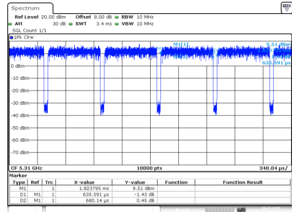
802.11n40_5310MHz_Chain 0
