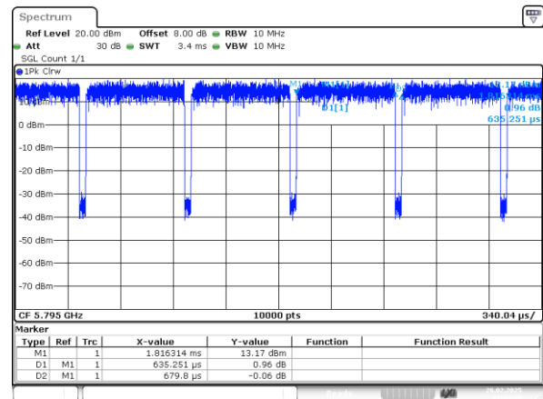
802.11n40_5795MHz_Chain 1
