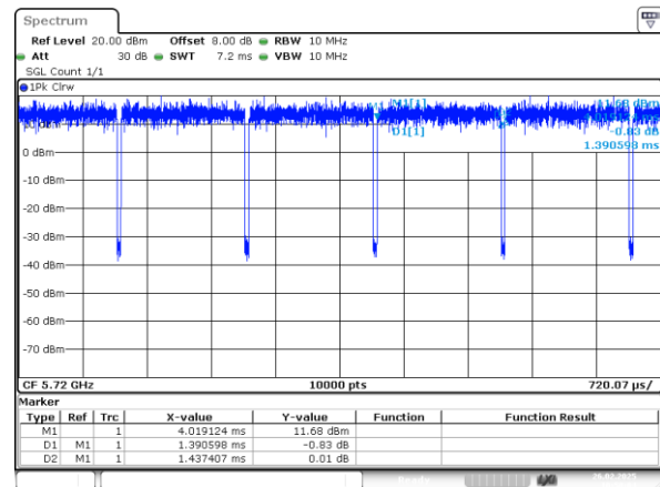
802.11a_5720MHz_Chain 0
