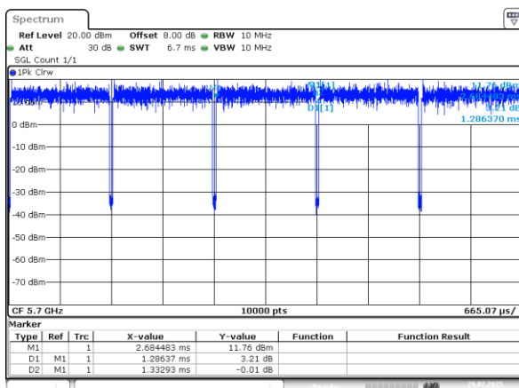
802.11n20_5700MHz_Chain 0
