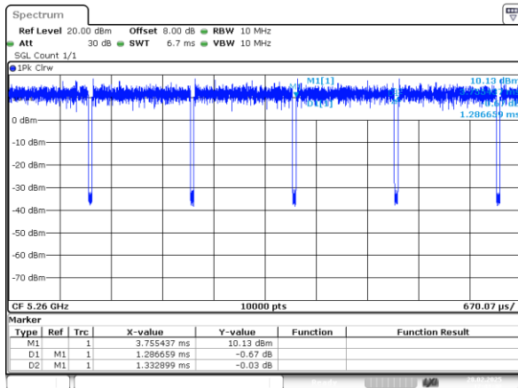
802.11n20_5260MHz_Chain 0
