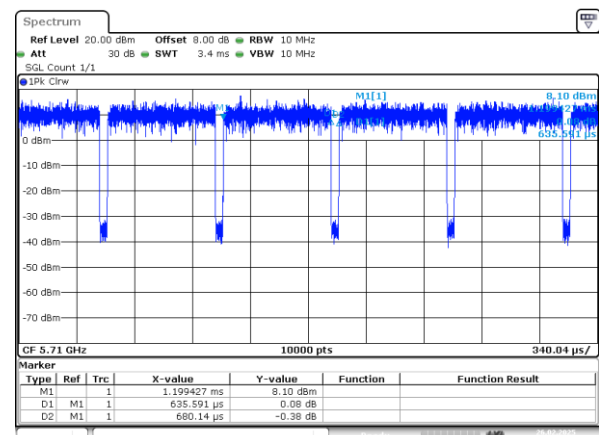
802.11n40_5710MHz_Chain 1
