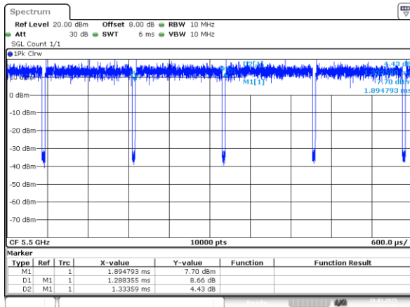
802.11n20_5500MHz_Chain 1
