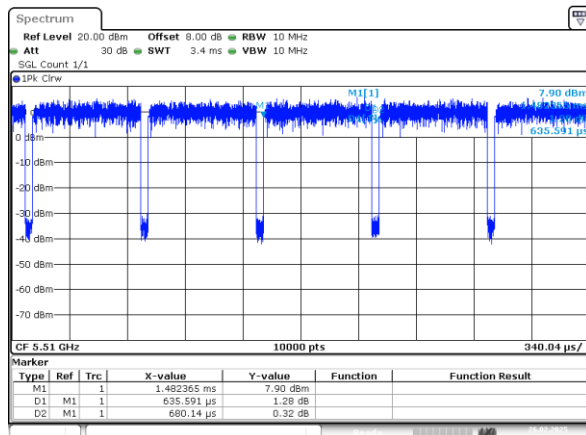
802.11n40_5510MHz_Chain 1
