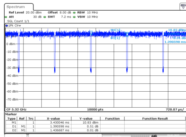
802.11a_5320MHz_Chain 1
