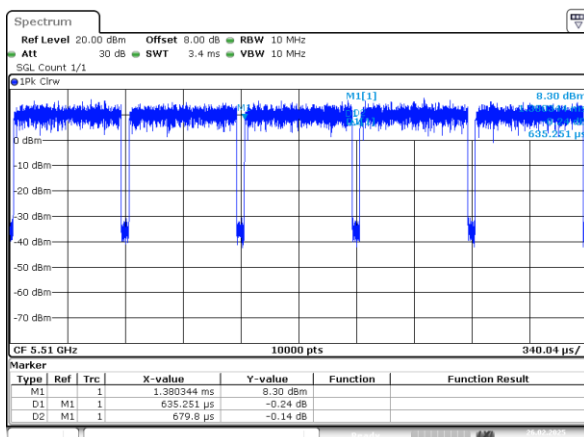
802.11n40_5510MHz_Chain 0
