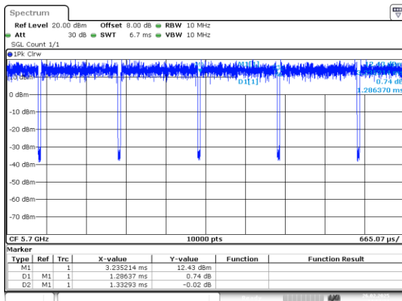
802.11n20_5700MHz_Chain 1
