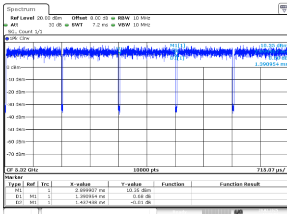
802.11a_5320MHz_Chain 0
