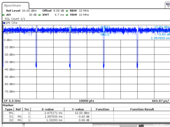
802.11n20_5500MHz_Chain 0
