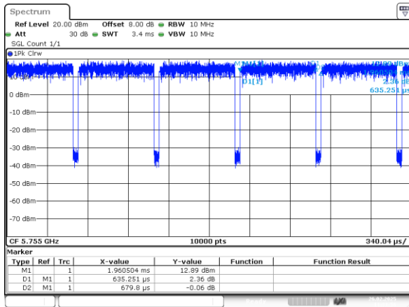
802.11n40_5755MHz_Chain 0
