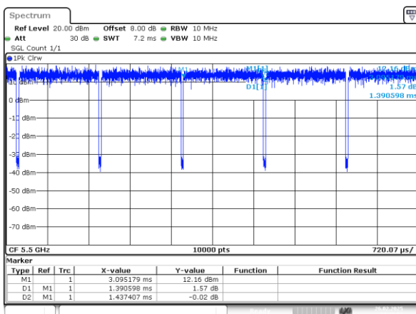
802.11a_5500MHz_Chain 1
