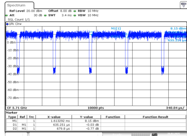
802.11n40_5710MHz_Chain 0
