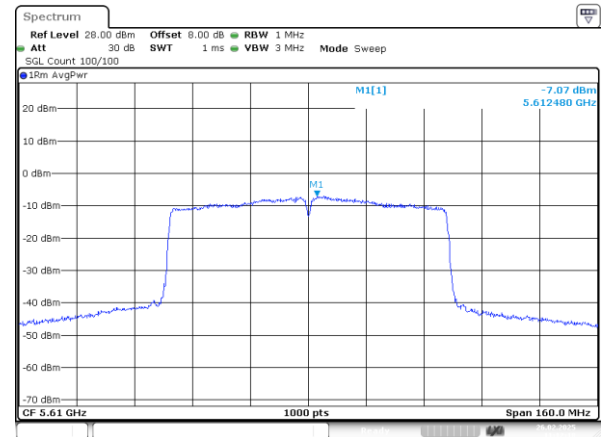
802.11ac80_5610MHz_Chain 0
