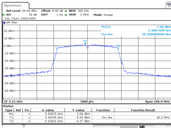
802.11n40_5510MHz_Chain 1
