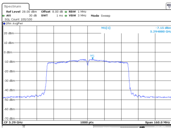
802.11ac80_5290MHz_Chain 0
