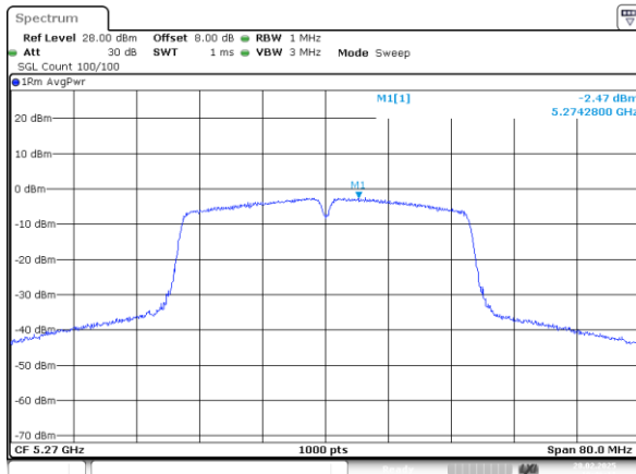
802.11n40_5270MHz_Chain 1
