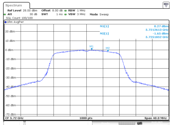
802.11a_5720MHz_Chain 0
