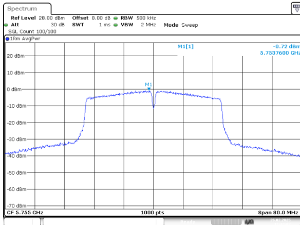
802.11n40_5755MHz_Chain 1
