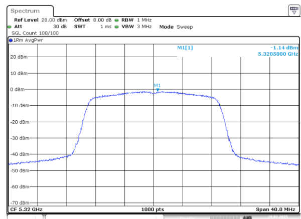
802.11n20_5320MHz_Chain 1
