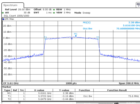
802.11ac80_5610MHz_Chain 1
