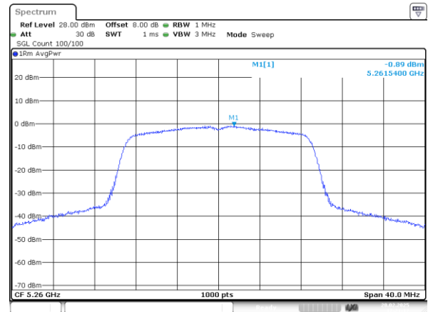
802.11n20_5260MHz_Chain 1
