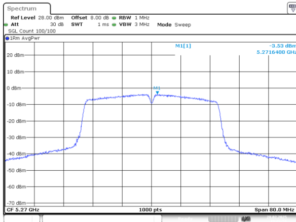
802.11n40_5270MHz_Chain 0
