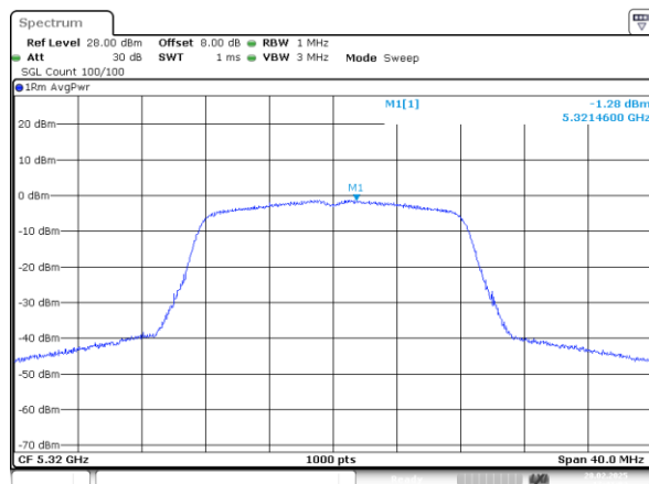
802.11a_5320MHz_Chain 0
