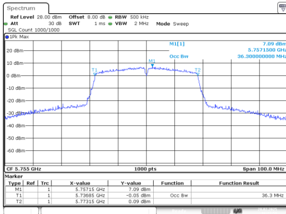
802.11n40_5755MHz_Chain 0
