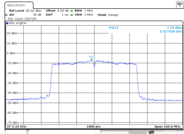
802.11ac80_5530MHz_Chain 1
