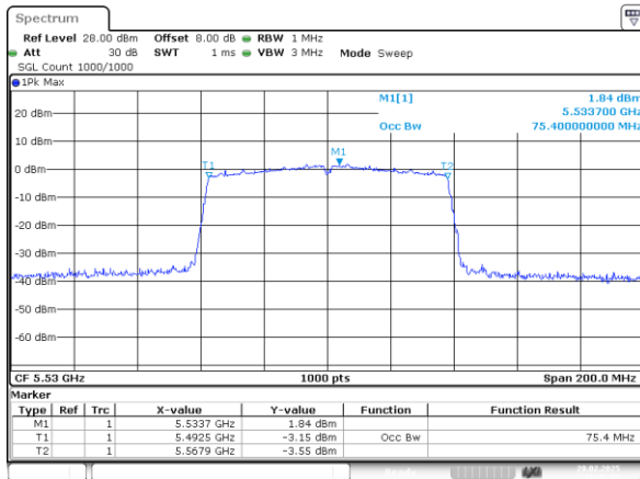
802.11ac80_5530MHz_Chain 0
