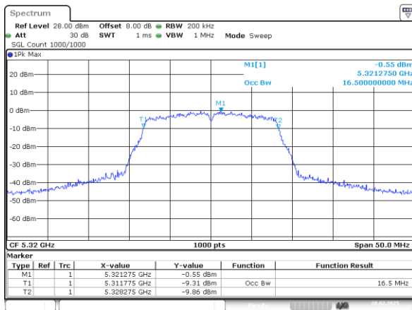
802.11a_5320MHz_Chain 0
