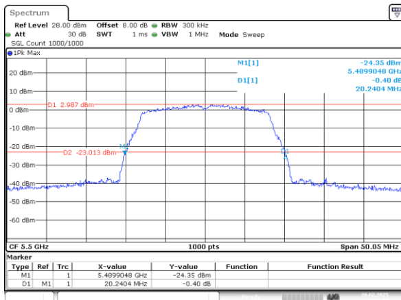
802.11a_5500MHz_Chain 1
