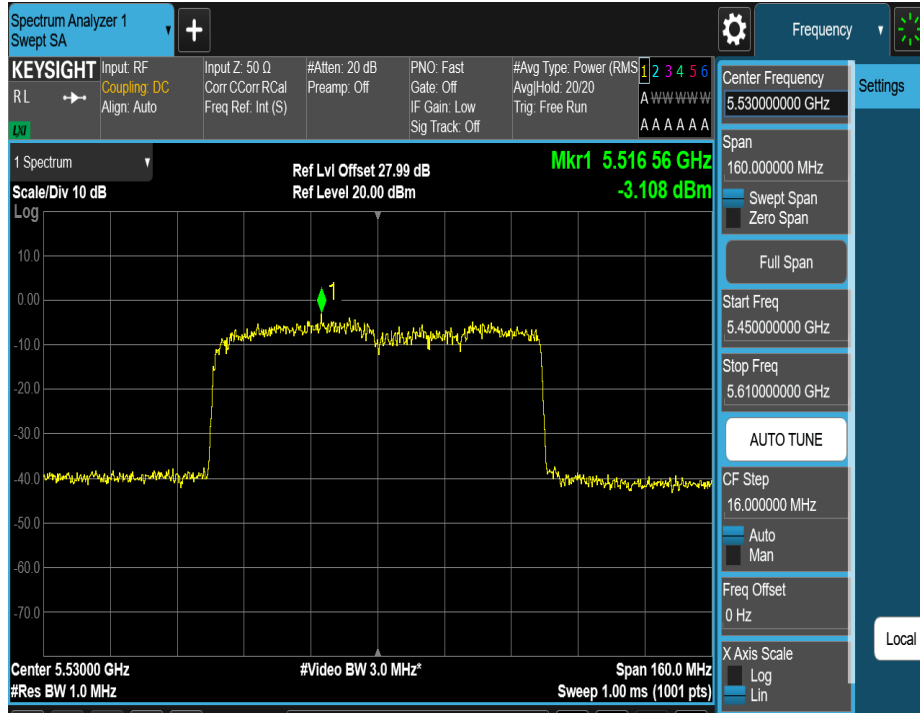
11AX80MIMO_Ant2_5530
