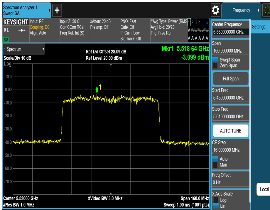
11AX80MIMO_Ant2_5530
