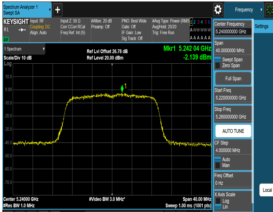
11AC20MIMO_Ant2_5240
