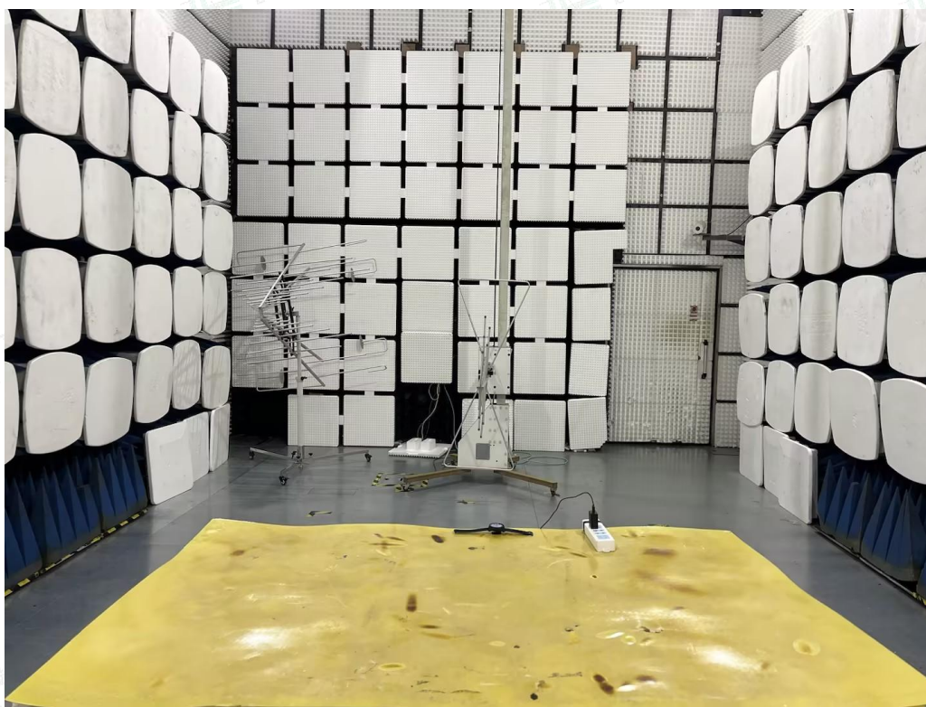
Fig. 2 (30MHz~1GHz)
