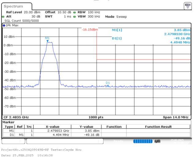
DH1_Hopping_Upper
