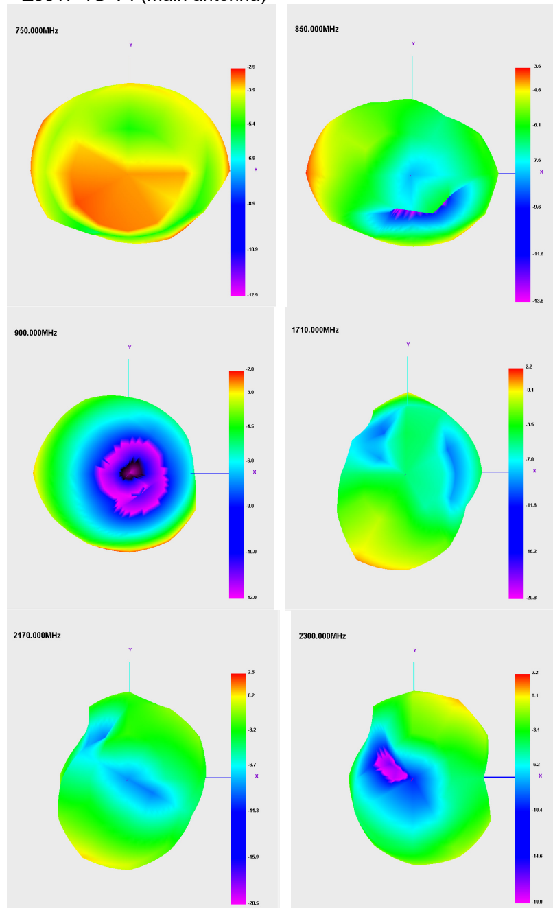
Z5517-4G-V4 (main antenna)
