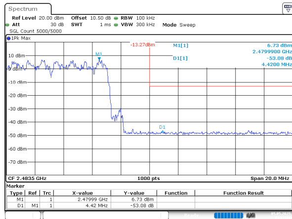
2EDR_DH1_Hopping_Upper
