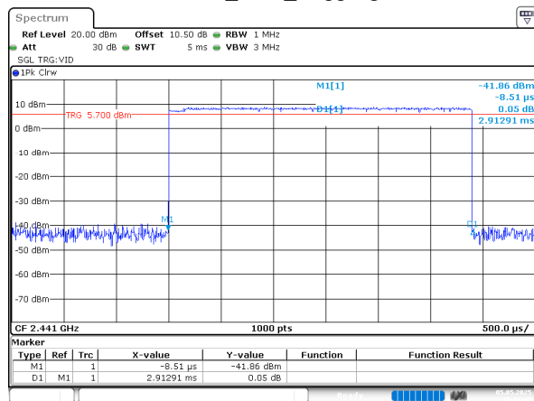
2EDR_DH5_Hopping
