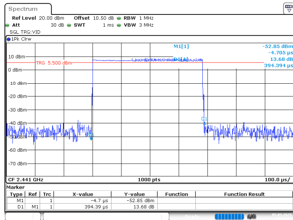
2EDR_DH1_Hopping
