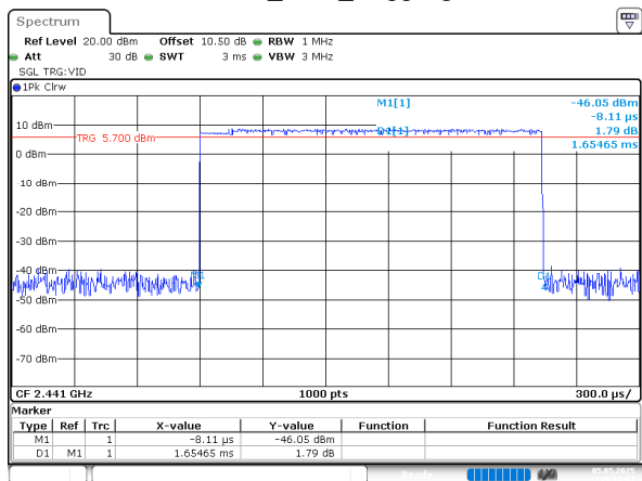
2EDR_DH3_Hopping
