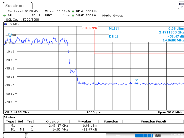
3EDR_DH1_Hopping_Upper
