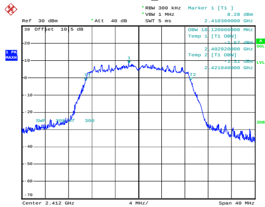
802.11n20_2412MHz
