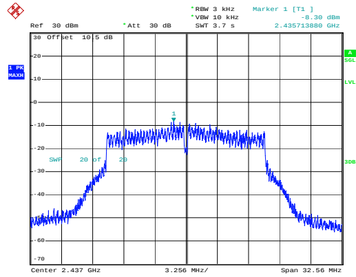
802.11g_2437MHz
