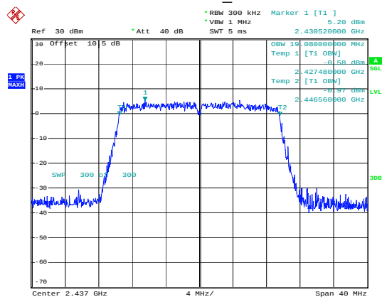
802.11ax20_2437MHz
