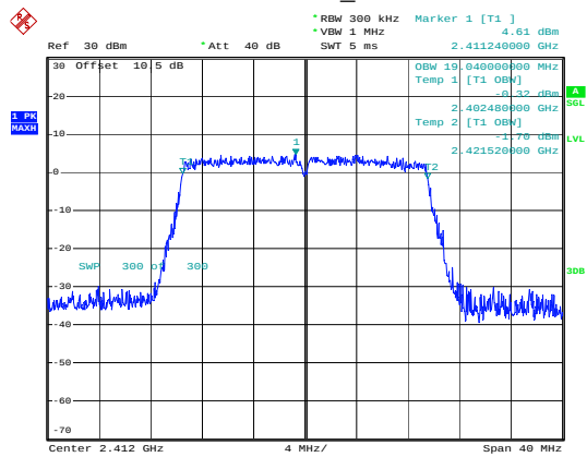
802.11ax20_2412MHz
