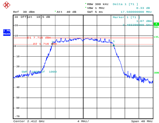
802.11n20_2412MHz
