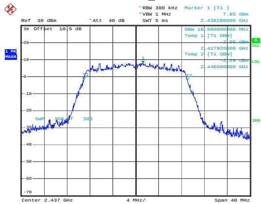
802.11n20_2437MHz
