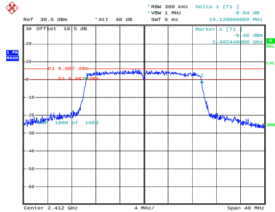
802.11ax20_2412MHz
