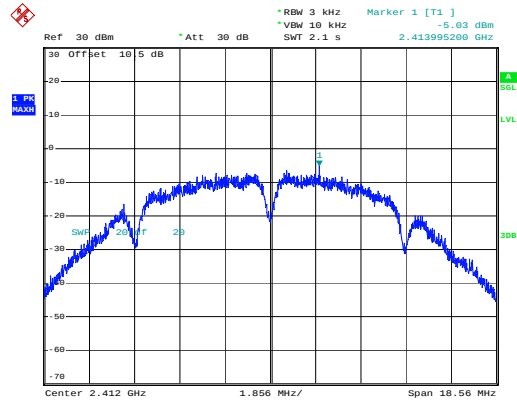
802.11b_2412MHz
