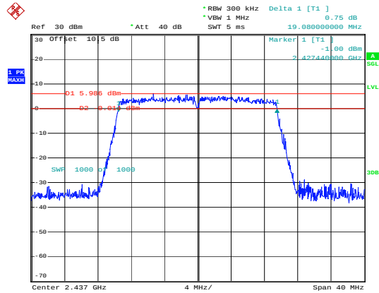
802.11ax20_2437MHz
