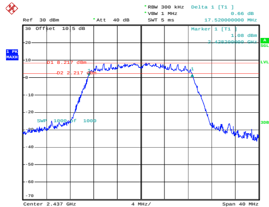
802.11n20_2437MHz
