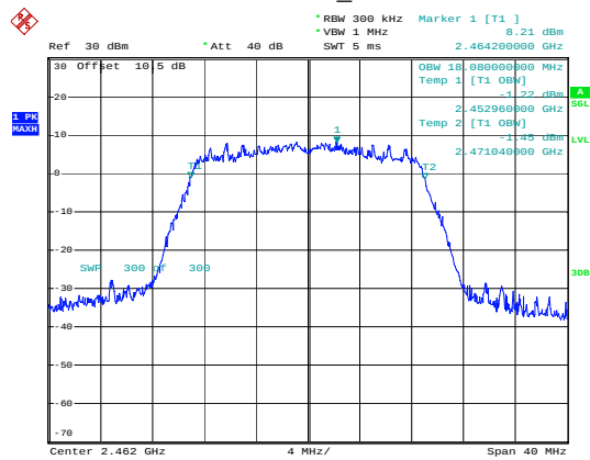
802.11n20_2462MHz
