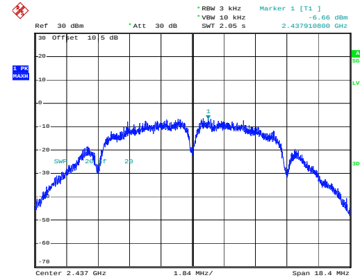
802.11b_2437MHz
