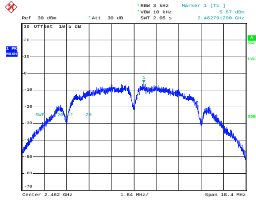
802.11b_2462MHz
