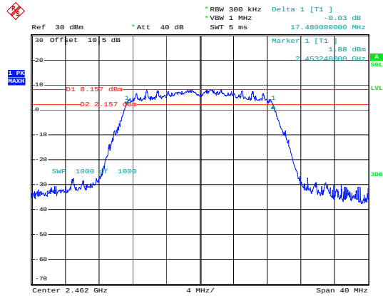
802.11n20_2462MHz
