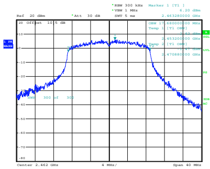
n20_2462MHz_Chain 0
