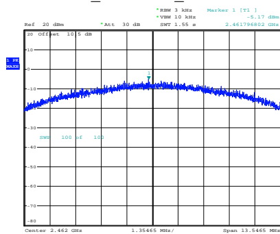
b_2462MHz_Chain 0
