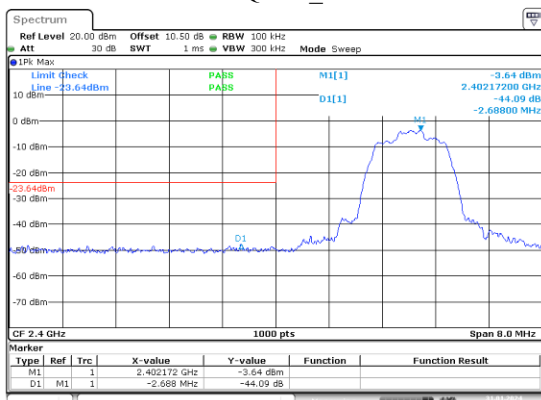
\pi/4 -DQPSK_Low
