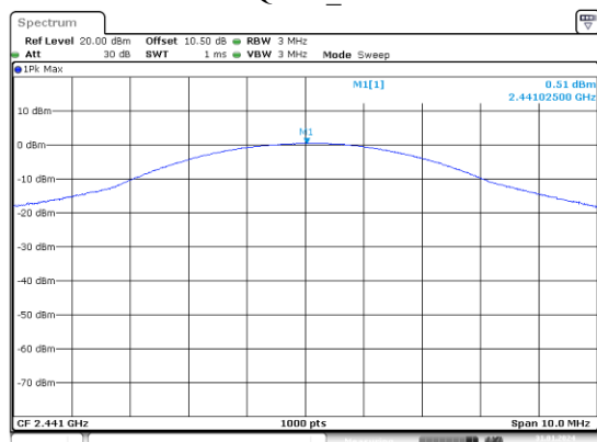
\pi/4 -DQPSK_Middle
