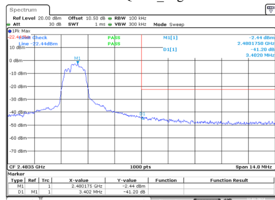
\pi/4 -DQPSK_High
