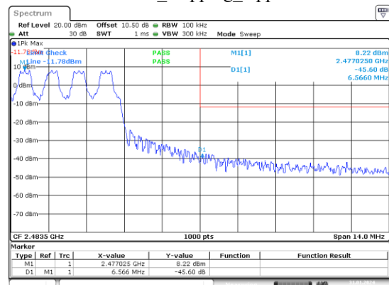
GFSK_Hopping_Upper
