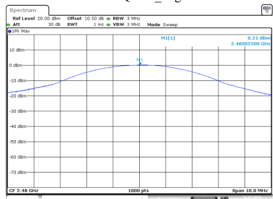
\pi/4 -DQPSK_High
