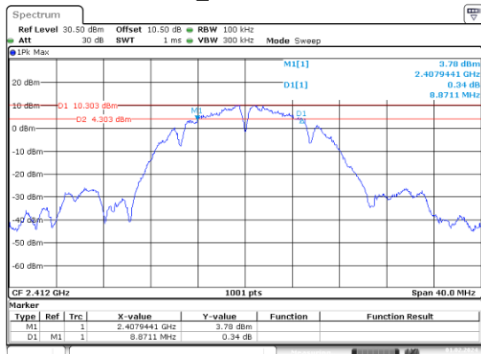
b_2412MHz
