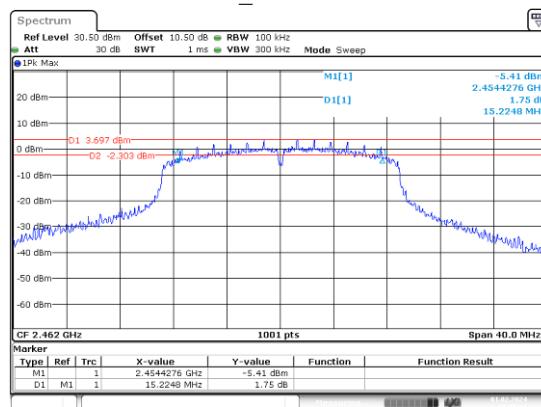
n20_2462MHz
