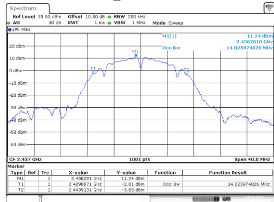
b_2437MHz
