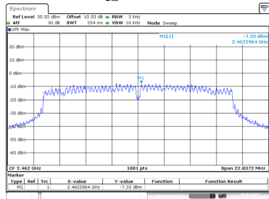
g_2462MHz
