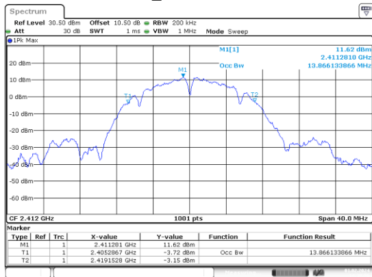
b_2412MHz
