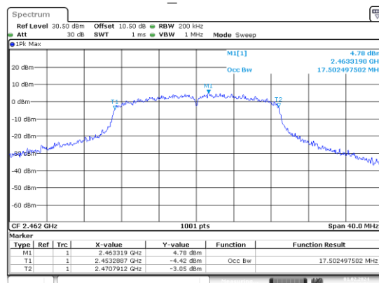
n20_2462MHz
