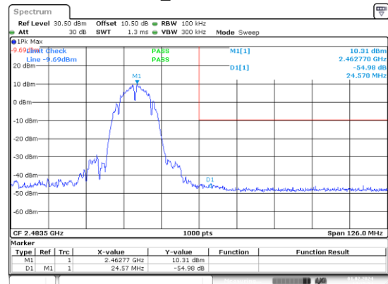
b_2462MHz
