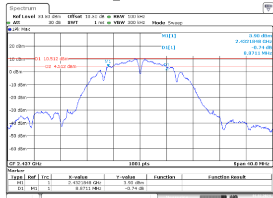
b_2437MHz
