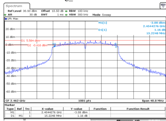
g_2462MHz
