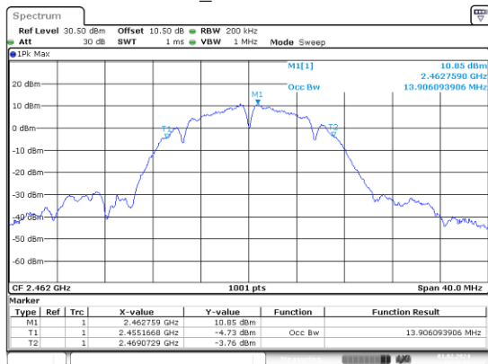
b_2462MHz
