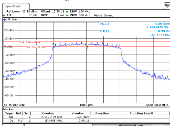
g_2437MHz
