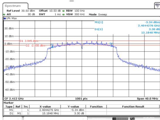
n20_2412MHz
