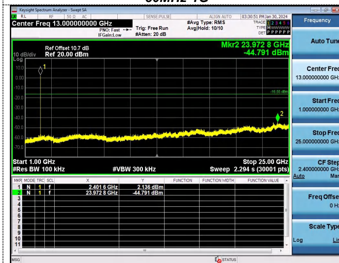
1G-25G
