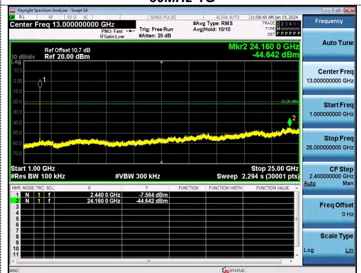
1G-25G
