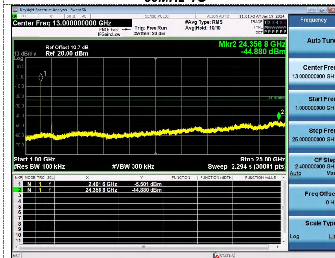
1G-25G
