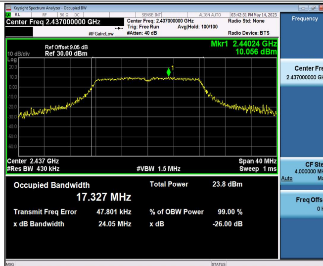
11G_Ant1_2437
