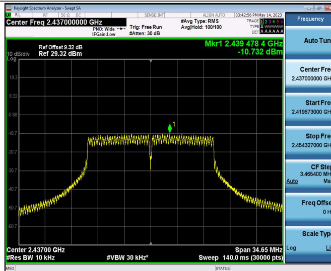
11G_Ant1_2437
