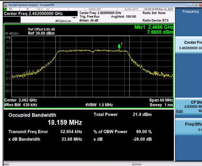
11N20SISO_Ant1_2462
