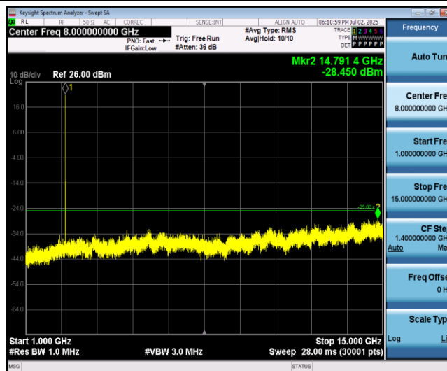
Band41-10MHz-QPSK-40290-1RB#0-Range2:1000~15000MHz
