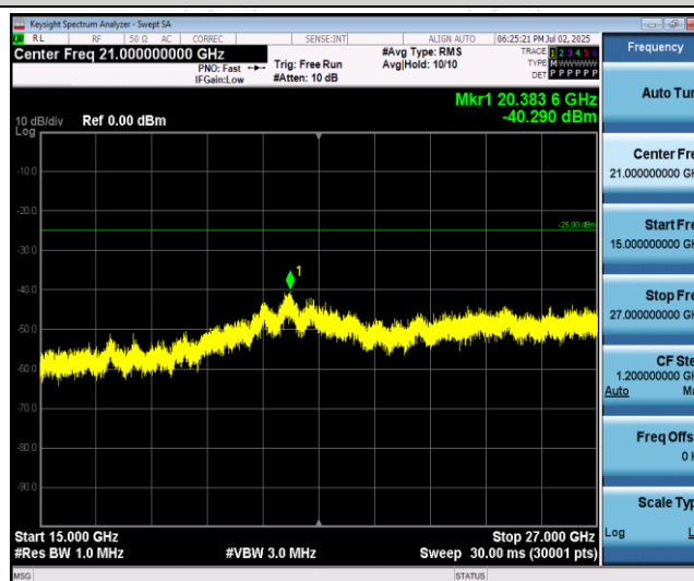
Band41-20MHz-QPSK-41140-1RB#0-Range3:15000~27000MHz
