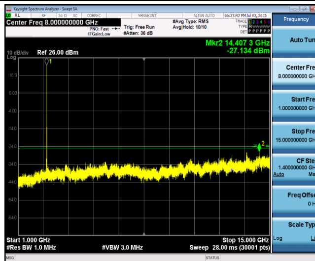
Band41-20MHz-QPSK-40690-1RB#0-Range2:1000~15000MHz
