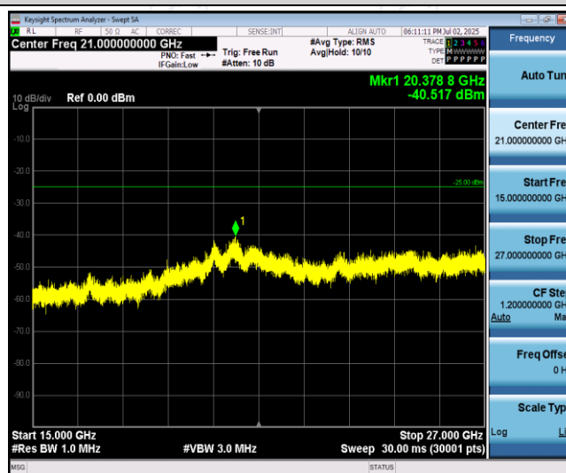
Band41-10MHz-QPSK-40290-1RB#0-Range3:15000~27000MHz
