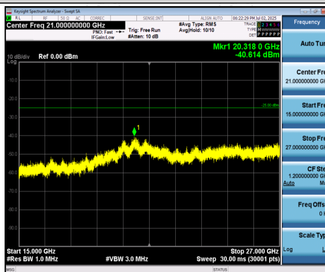
Band41-20MHz-QPSK-40340-1RB#0-Range3:15000~27000MHz
