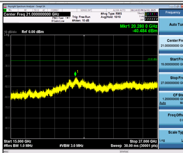
Band41-10MHz-QPSK-41190-1RB#0-Range3:15000~27000MHz
