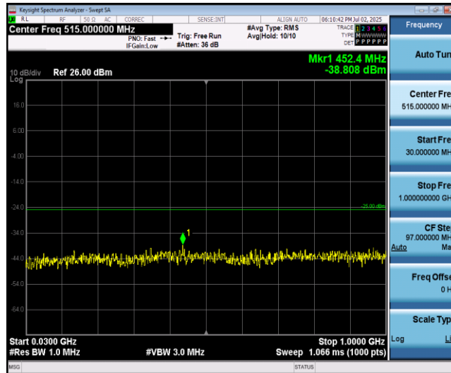
Band41-10MHz-QPSK-40290-1RB#0-Range1:30~1000MHz
