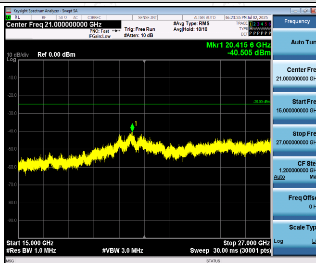
Band41-20MHz-QPSK-40690-1RB#0-Range3:15000~27000MHz
