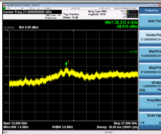
Band41-10MHz-QPSK-40690-1RB#0-Range3:15000~27000MHz
