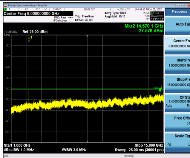
Band41-5MHz-QPSK-41215-1RB#0-Range2:1000~15000MHz
