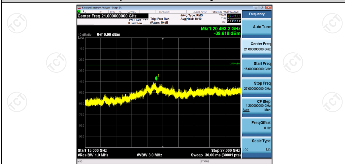
Band41-5MHz-QPSK-40265-1RB#0-Range3:15000~27000MHz
