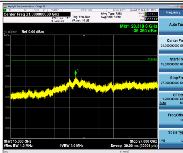
Band41-5MHz-QPSK-41215-1RB#0-Range3:15000~27000MHz
