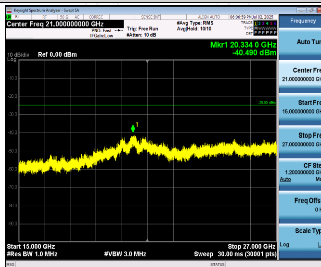
Band41-5MHz-QPSK-40690-1RB#0-Range3:15000~27000MHz
