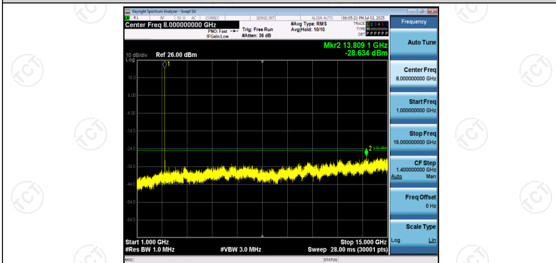
Band41-5MHz-QPSK-40265-1RB#0-Range2:1000~15000MHz
