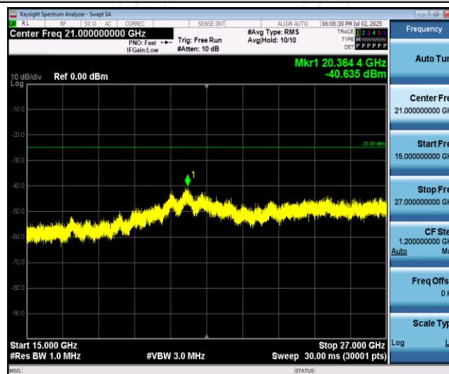
Band7-20MHz-QPSK-21100-1RB#0-Range3:15000~27000MHz
