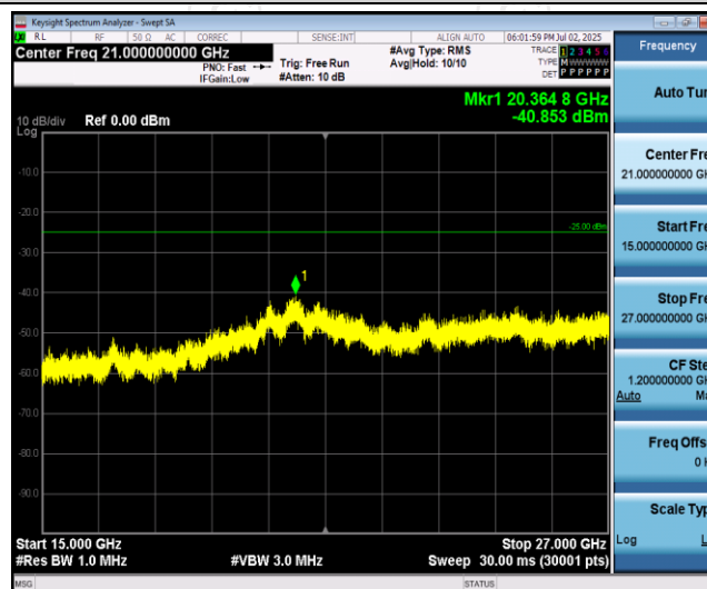
Band7-20MHz-QPSK-21350-1RB#0-Range3:15000~27000MHz
