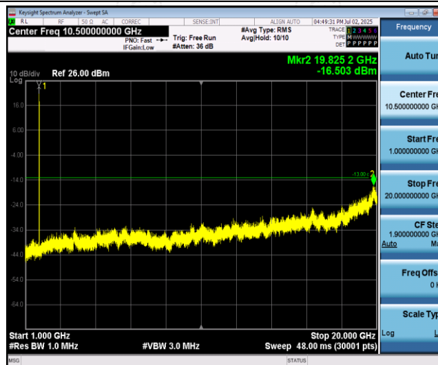
Band4-3MHz-QPSK-20385-1RB#0-Range2:1000~20000MHz
