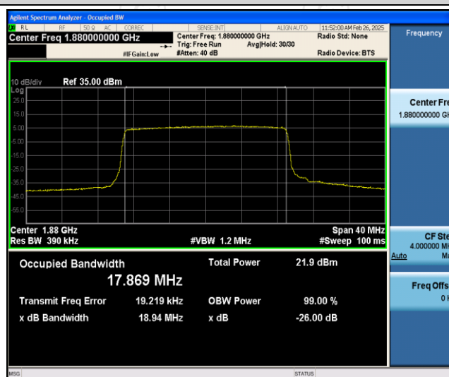
Band2-20MHz-16QAM-18900-100RB#0
