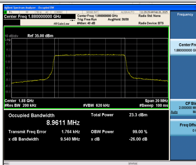
Band2-10MHz-QPSK-18900-50RB#0
