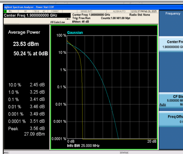
Band2-20MHz-QPSK-19100-1RB#0
