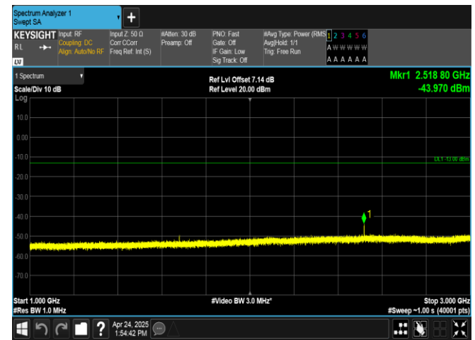
Band26(824-849)-10MHz-QPSK-26990-1RB#0-1000~3000-PASS
