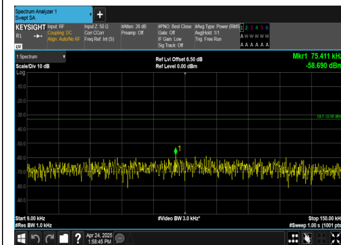
Band26(824-849)-10MHz-QPSK-26990-50RB#0-0.009~0.15-PASS
