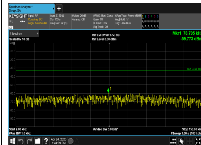
Band26(824-849)-10MHz-QPSK-26840-50RB#0-0.009~0.15-PASS
