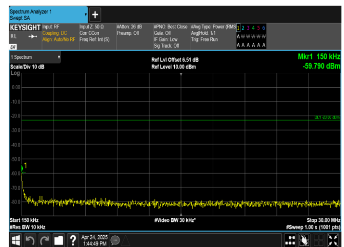
Band26(824-849)-10MHz-QPSK-26840-50RB#0-0.15~30-PASS
