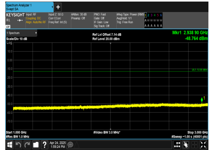
Band26(824-849)-10MHz-QPSK-26990-50RB#0-1000~3000-PASS
