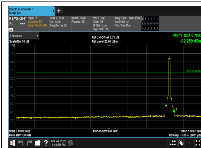
Band26(824-849)-10MHz-QPSK-26840-50RB#0-30~1000-PASS
