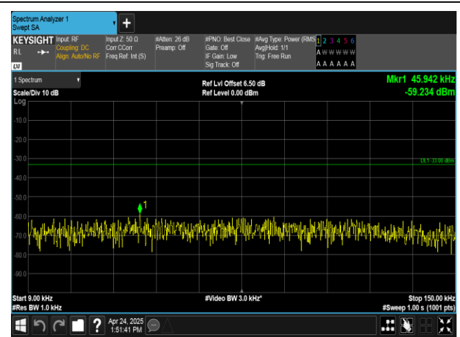
Band26(824-849)-10MHz-QPSK-26915-50RB#0-0.009~0.15-PASS
