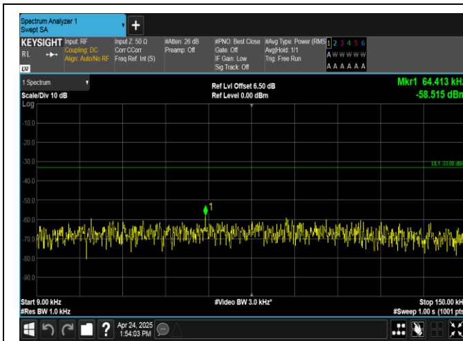
Band26(824-849)-10MHz-QPSK-26990-1RB#0-0.009~0.15-PASS
