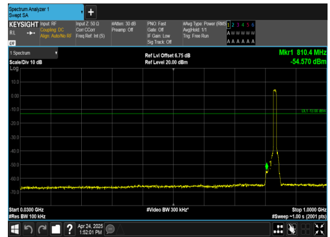
Band26(824-849)-10MHz-QPSK-26915-50RB#0-30~1000-PASS
