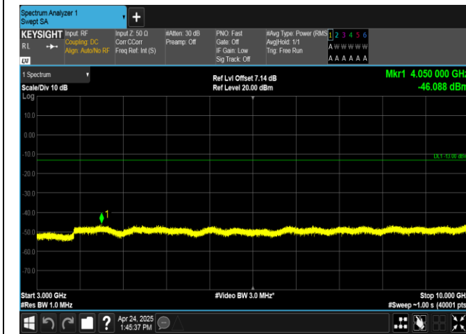
Band26(824-849)-10MHz-QPSK-26840-50RB#0-3000~10000-PASS
