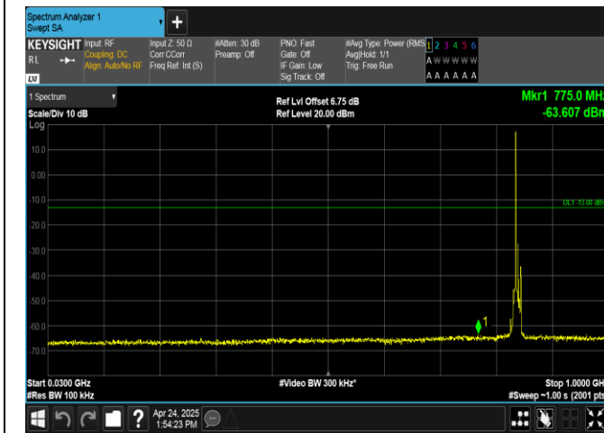
Band26(824-849)-10MHz-QPSK-26990-1RB#0-30~1000-PASS
