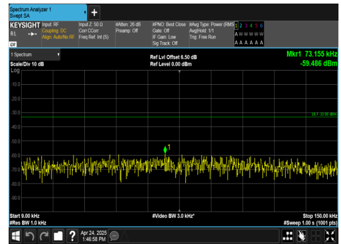
Band26(824-849)-10MHz-QPSK-26915-1RB#0-0.009~0.15-PASS
