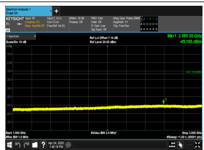
Band26(824-849)-10MHz-QPSK-26840-50RB#0-1000~3000-PASS
