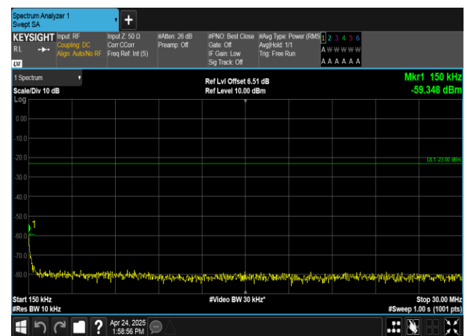
Band26(824-849)-10MHz-QPSK-26990-50RB#0-0.15~30-PASS
