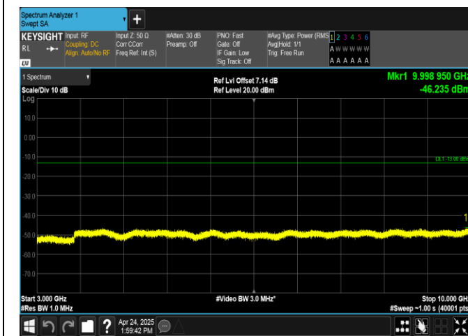
Band26(824-849)-10MHz-QPSK-26990-50RB#0-3000~10000-PASS
