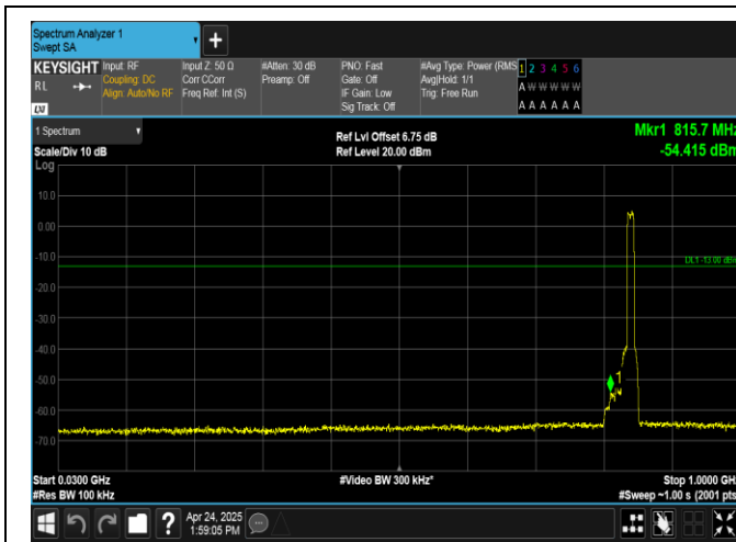
Band26(824-849)-10MHz-QPSK-26990-50RB#0-30~1000-PASS
