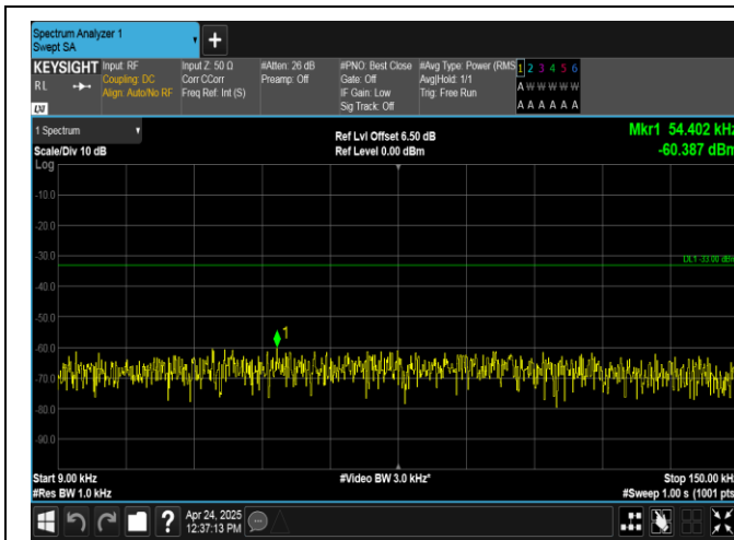
Band26(824-849)-3MHz-QPSK-27025-1RB#0-0.009~0.15-PASS
