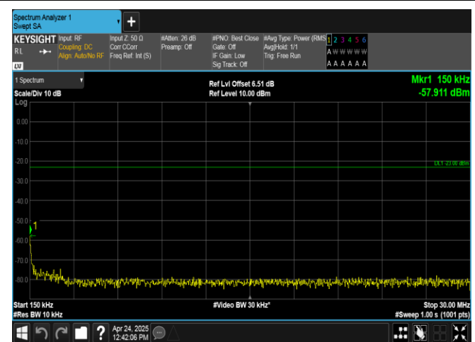
Band26(824-849)-3MHz-QPSK-27025-15RB#0-0.15~30-PASS
