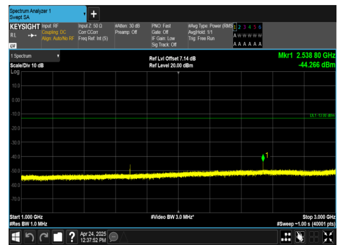
Band26(824-849)-3MHz-QPSK-27025-1RB#0-1000~3000-PASS
