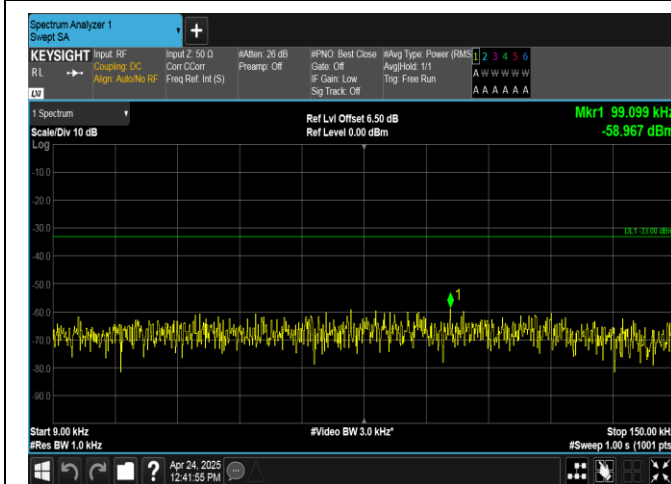
Band26(824-849)-3MHz-QPSK-27025-15RB#0-0.009~0.15-PASS
