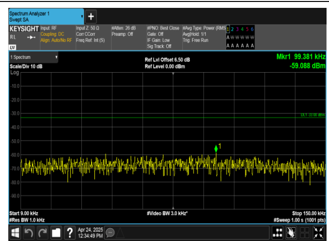
Band26(824-849)-3MHz-QPSK-26915-15RB#0-0.009~0.15-PASS
