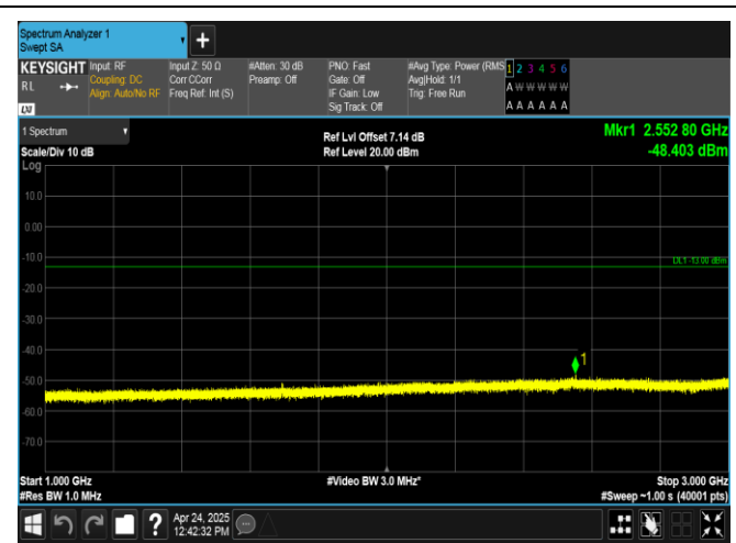
Band26(824-849)-3MHz-QPSK-27025-15RB#0-1000~3000-PASS
