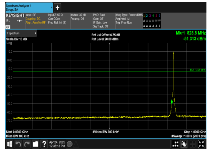
Band26(824-849)-3MHz-QPSK-26915-15RB#0-30~1000-PASS
