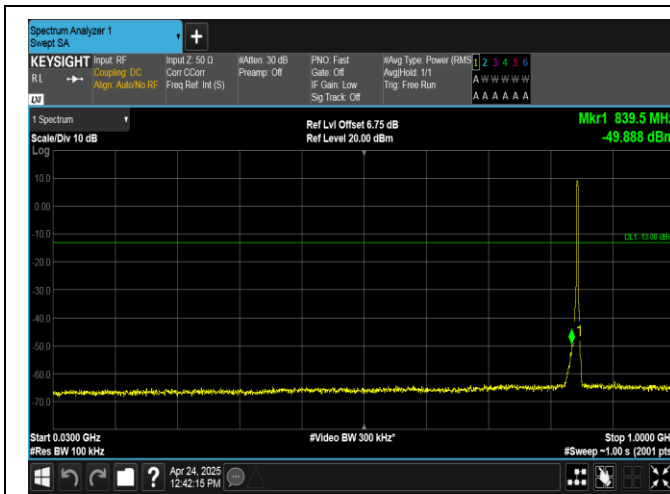
Band26(824-849)-3MHz-QPSK-27025-15RB#0-30~1000-PASS
