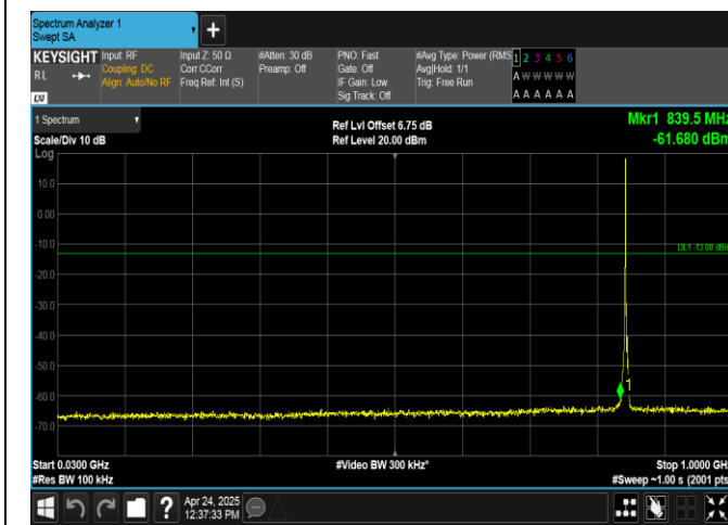
Band26(824-849)-3MHz-QPSK-27025-1RB#0-30~1000-PASS
