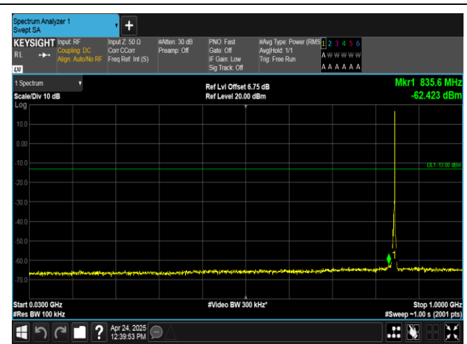
Band26(824-849)-3MHz-QPSK-27025-1RB#14-30~1000-PASS
