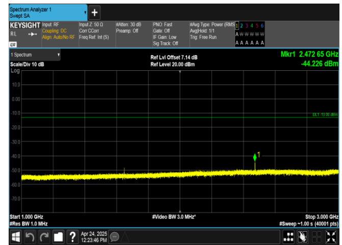
Band26(824-849)-3MHz-QPSK-26805-1RB#0-1000~3000-PASS
