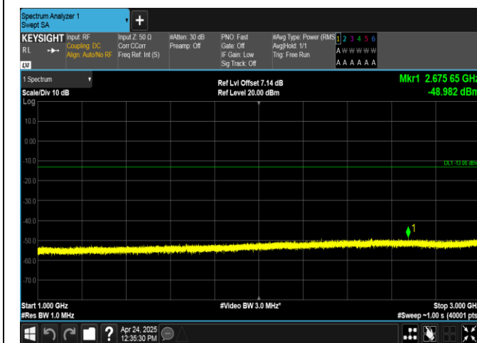
Band26(824-849)-3MHz-QPSK-26915-15RB#0-1000~3000-PASS
