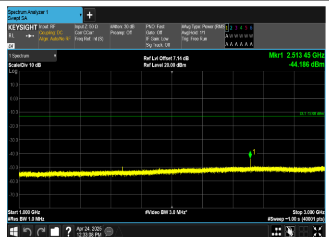
Band26(824-849)-3MHz-QPSK-26915-1RB#14-1000~3000-PASS
