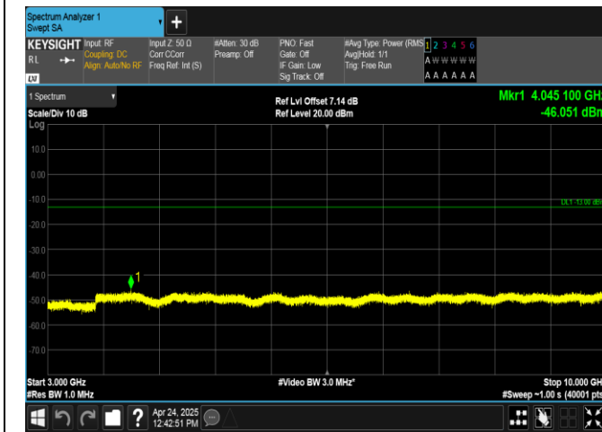
Band26(824-849)-3MHz-QPSK-27025-15RB#0-3000~10000-PASS
