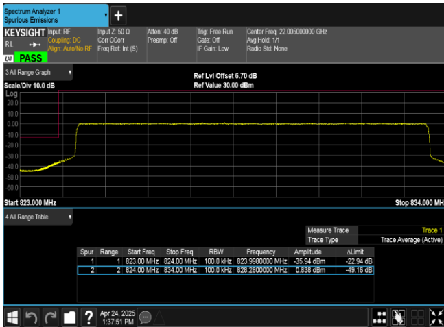
Band26(824-849)-10MHz-QPSK-26840-50RB#0-PASS
