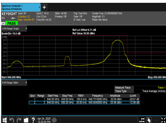
Band26(824-849)-3MHz-QPSK-27025-1RB#14-PASS
