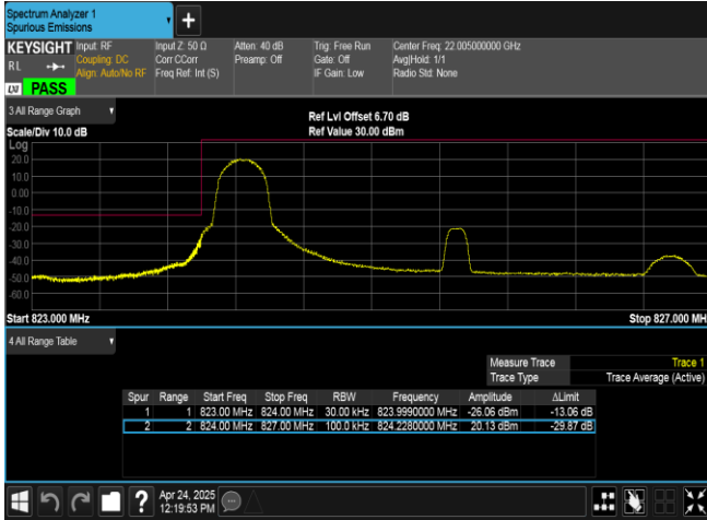
Band26(824-849)-3MHz-QPSK-26805-1RB#0-PASS
