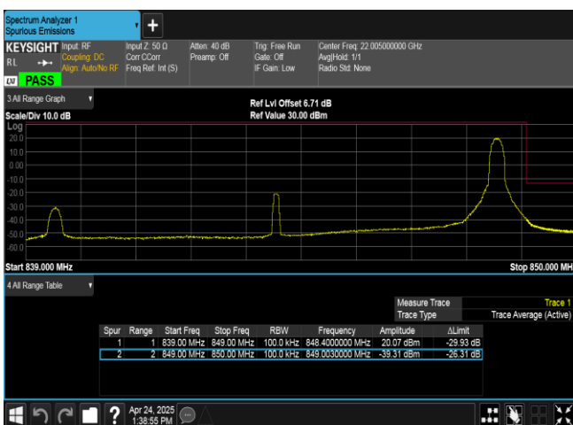
Band26(824-849)-10MHz-QPSK-26990-1RB#49-PASS
