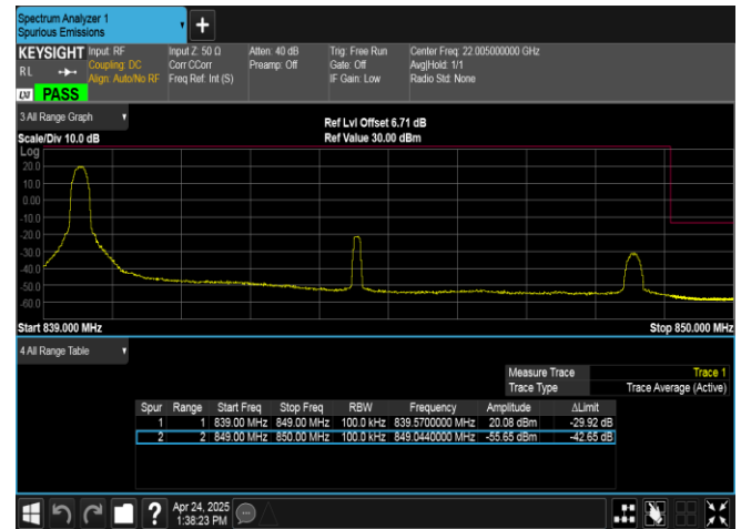
Band26(824-849)-10MHz-QPSK-26990-1RB#0-PASS
