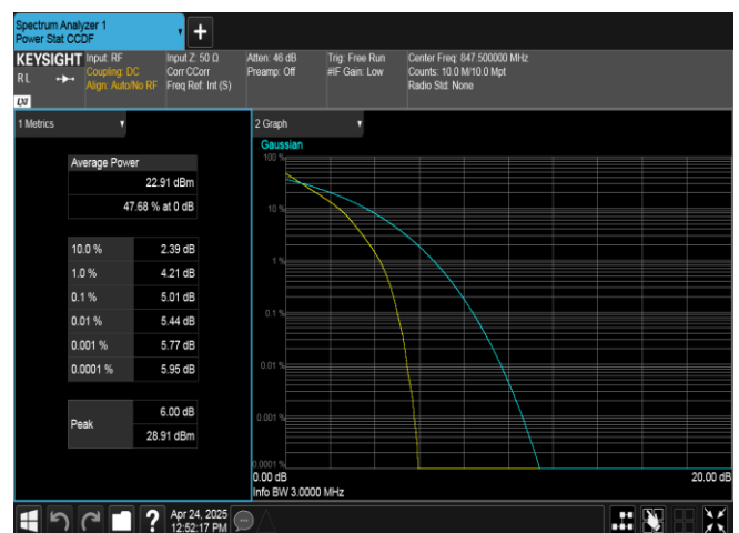
Band26(824-849)-3MHz-QPSK-27025-15RB#0-PASS
