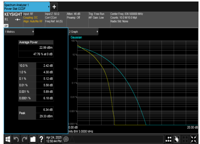
Band26(824-849)-3MHz-QPSK-26915-15RB#0-PASS
