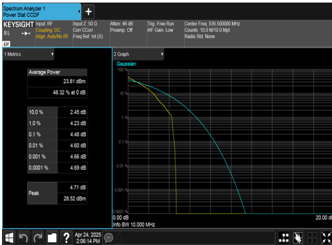
Band26(824-849)-10MHz-QPSK-26915-1RB#0-PASS
