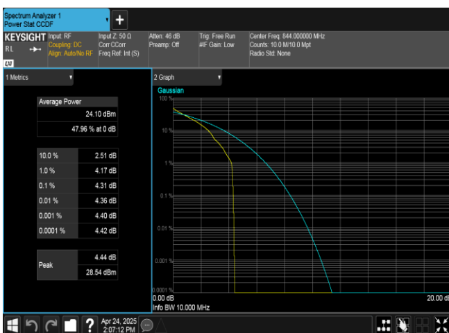
Band26(824-849)-10MHz-QPSK-26990-1RB#0-PASS
