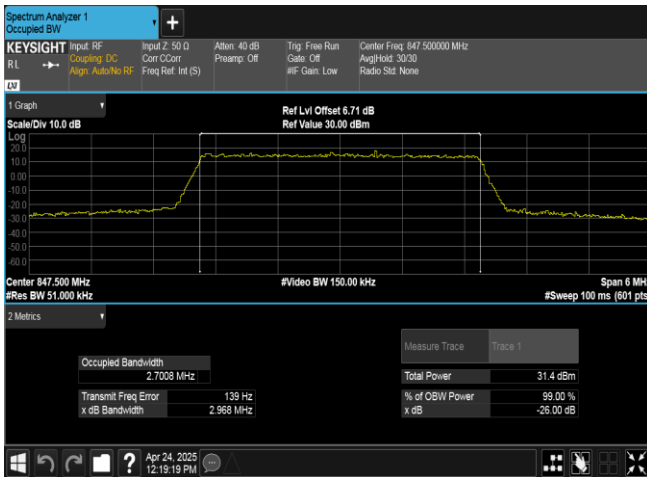
Band26(824-849)-3MHz-QPSK-27025-15RB#0-PASS
