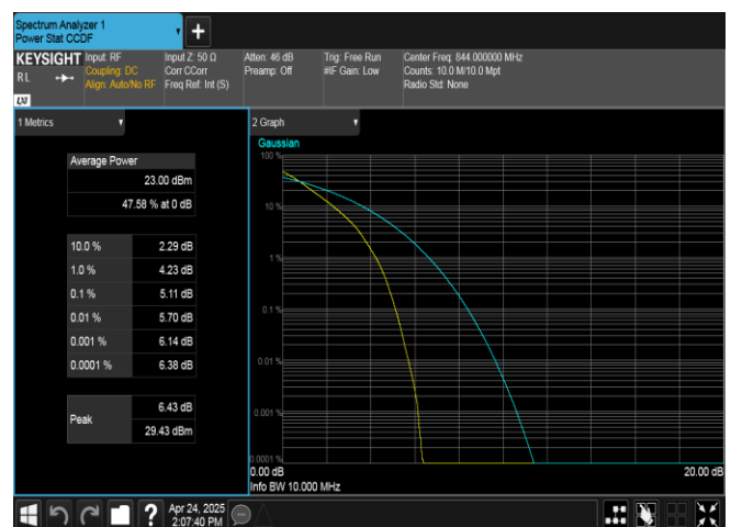
Band26(824-849)-10MHz-QPSK-26990-50RB#0-PASS
