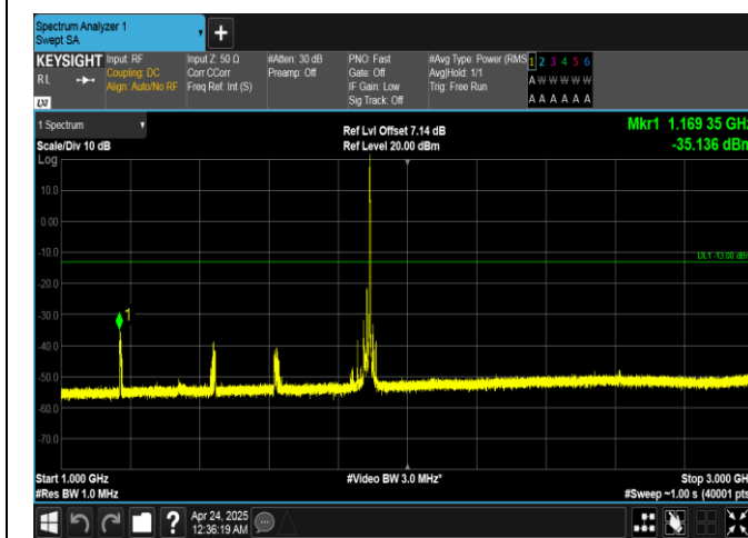
Band25-20MHz-16QAM-26365-1RB#99-1000~3000-PASS
