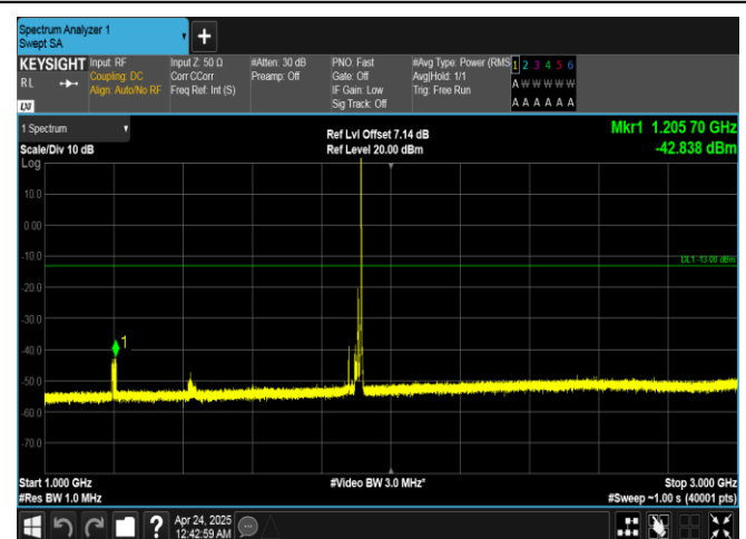
Band25-20MHz-16QAM-26590-1RB#99-1000~3000-PASS
